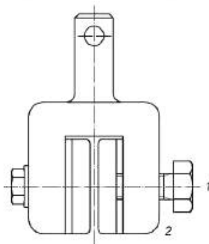
Рисунок 2 – Клиновый зажим
