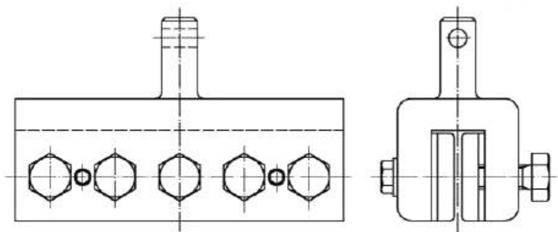
Рисунок 5 – Конструкция зажима, используемого для испытания георешеток
