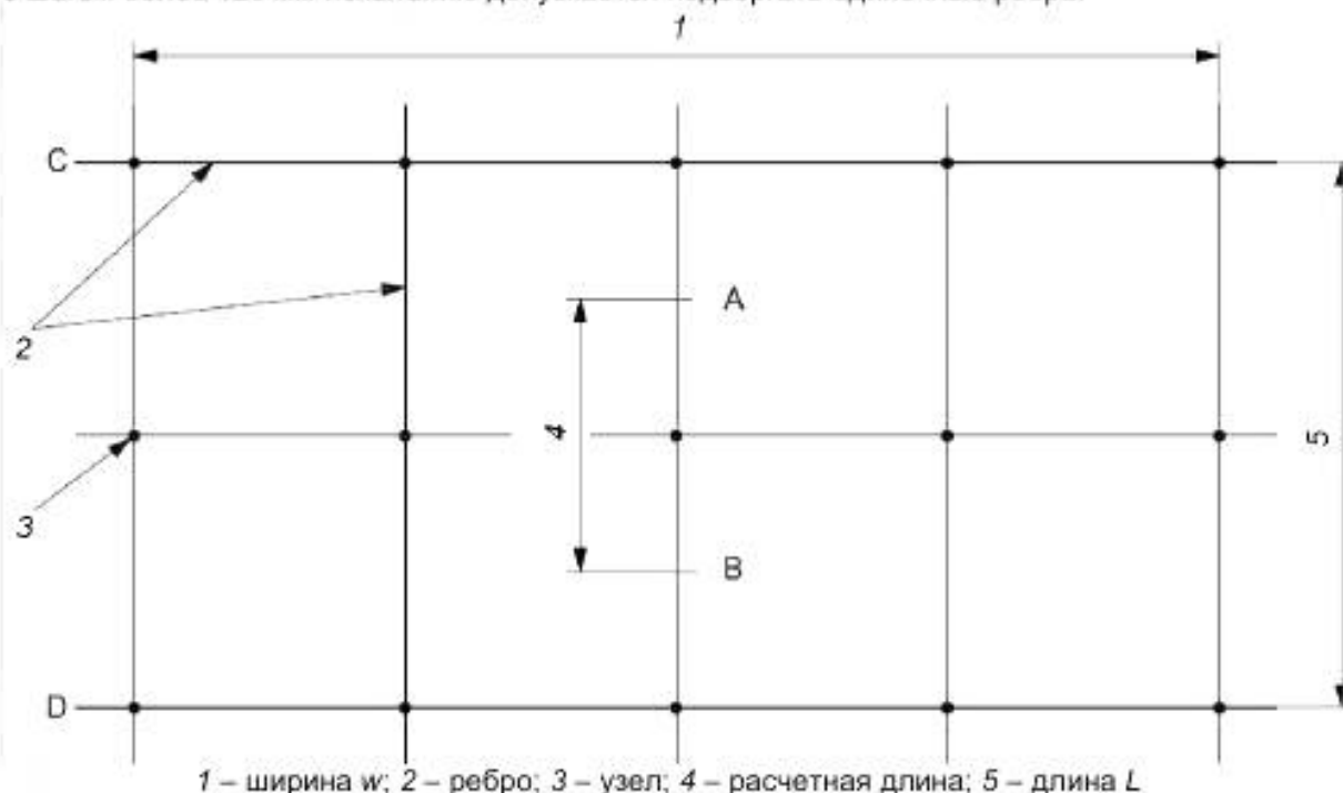
Рисунок 7 – Стандартная георешетка
