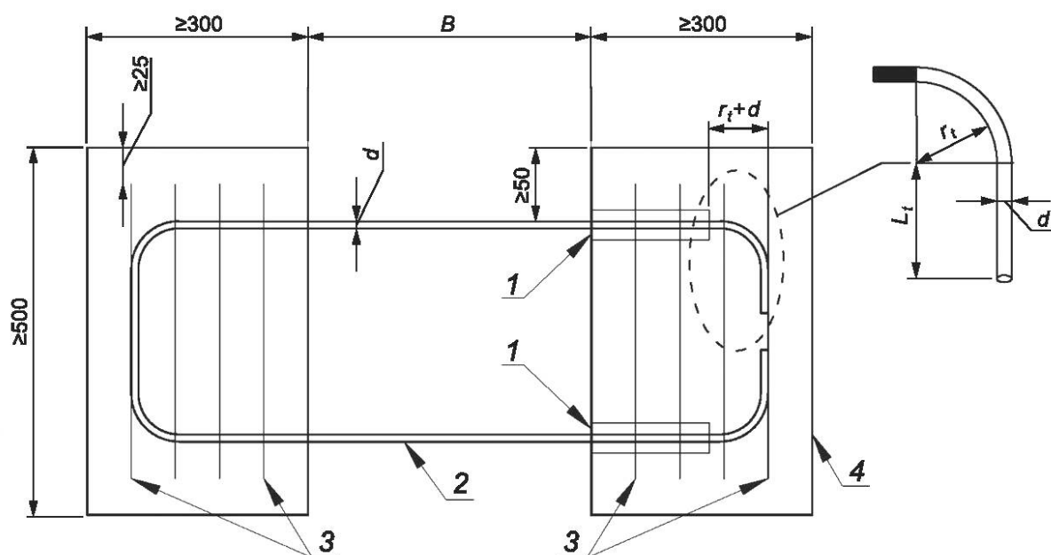
1 — поливинилхлоридный вкладыш или трубка; 2 — АКП; 3 — стальные хомуты (при наличии); 4 — бетонный блок
