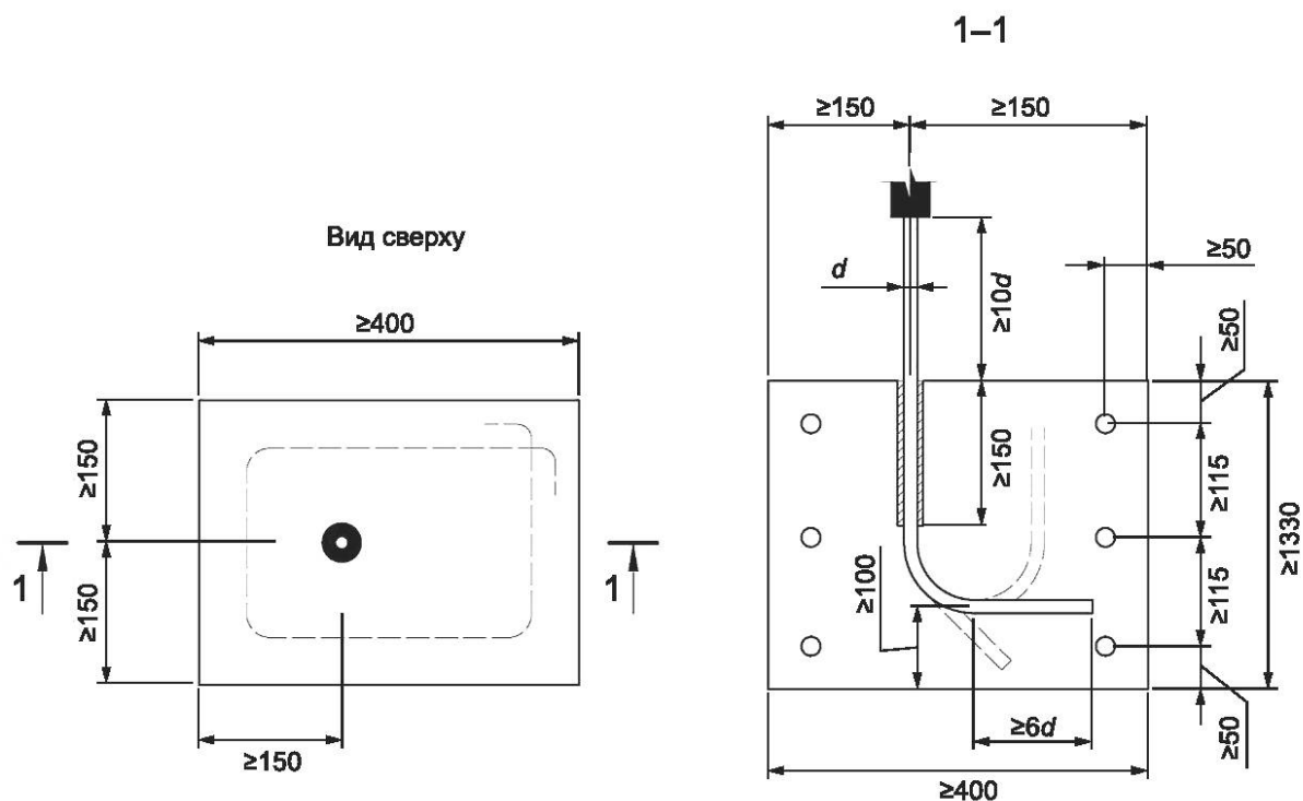
Рисунок 9.2 — Рекомендуемые размеры образца для испытаний
