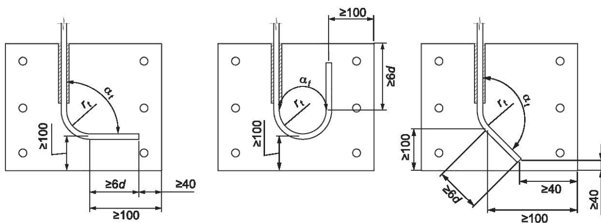
Рисунок 9.3 — Варианты образцов для испытаний с разным углом изгиба \alpha , стержня АКП
