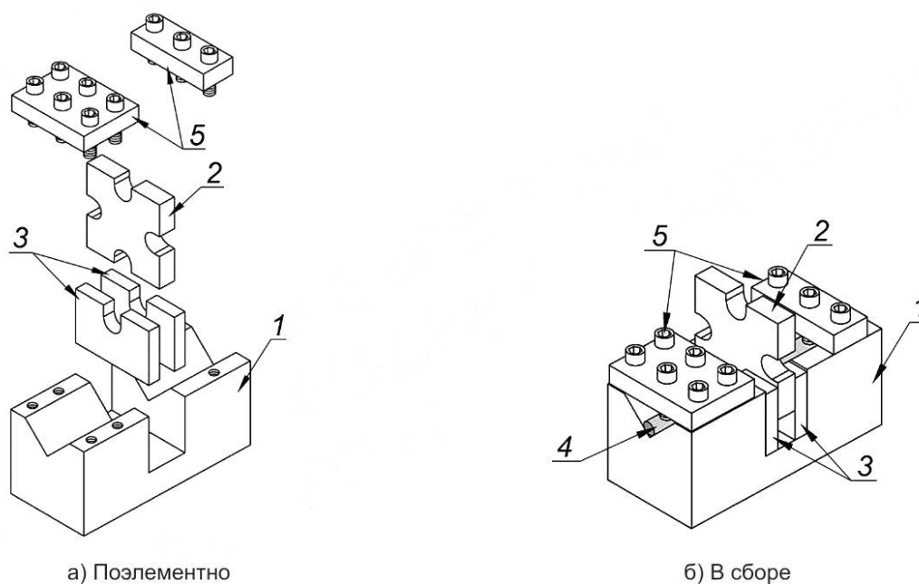
Рисунок 7.1 — Приспособление для испытания образцов на поперечный срез
