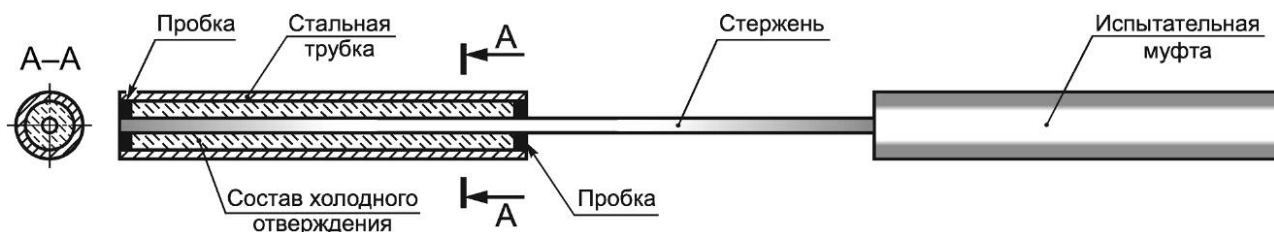
Рисунок 5.1 — Вид типового испытательного образца
