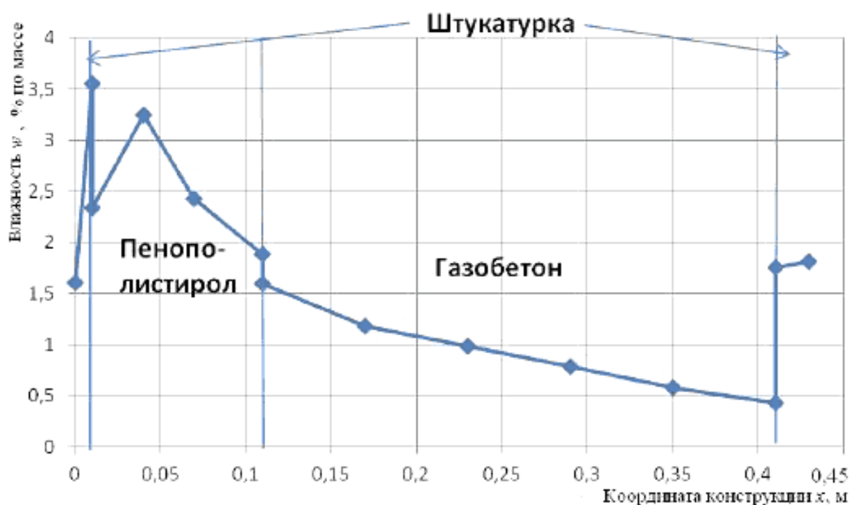
Рисунок Г.1 – Распределение влажности внутри конструкции
