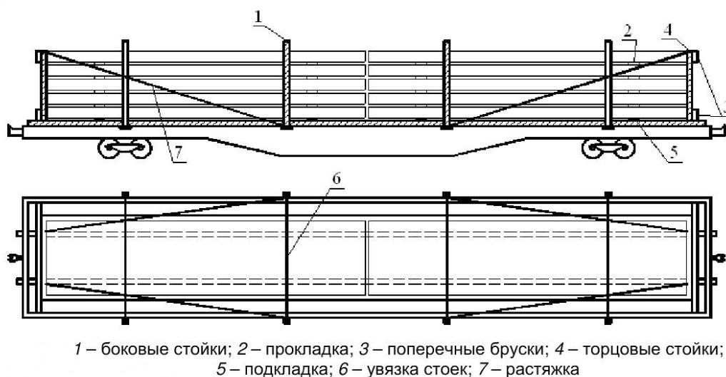
Рисунок 3 – Размещение и крепление железобетонных плит на платформе при перевозке их по железной дороге
