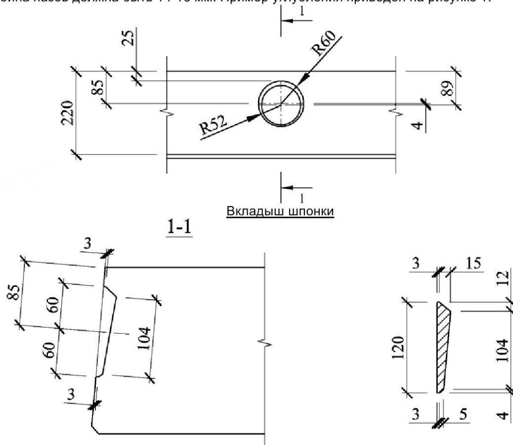
Рисунок 1 – Углубление на боковой поверхности плиты
