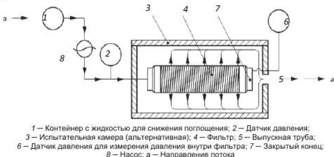
Рисунок В.1 – Стенд для испытания на прочность с альтернативной испытательной камерой
