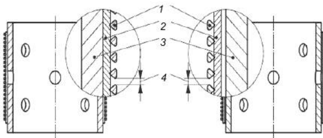
а) прямая намотка
