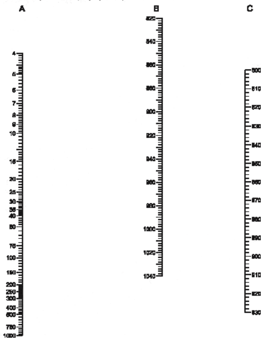
А — кинематическая вязкость при 50 °С, мм 2 /с; В — плотность при 15 °С, кг/м 3 ; С — ССАИ
