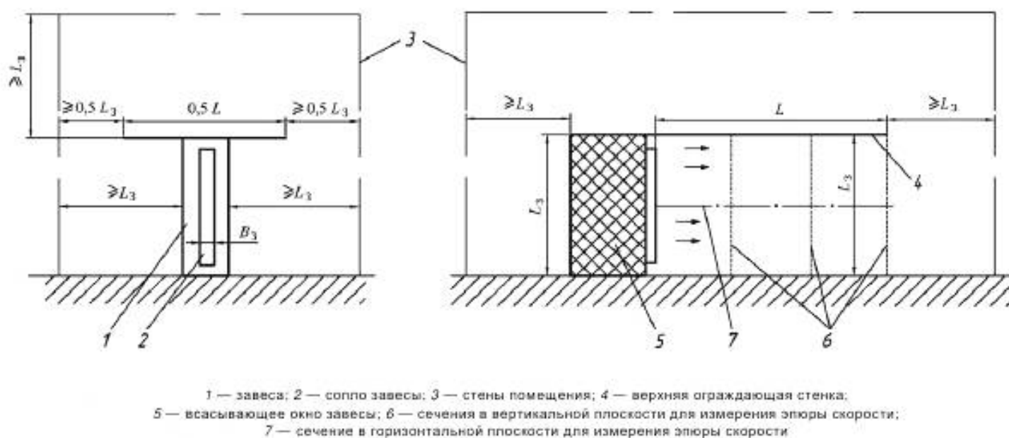
Рисунок А.1 — Схема стенда для определения максимальной скорости на оси струи
