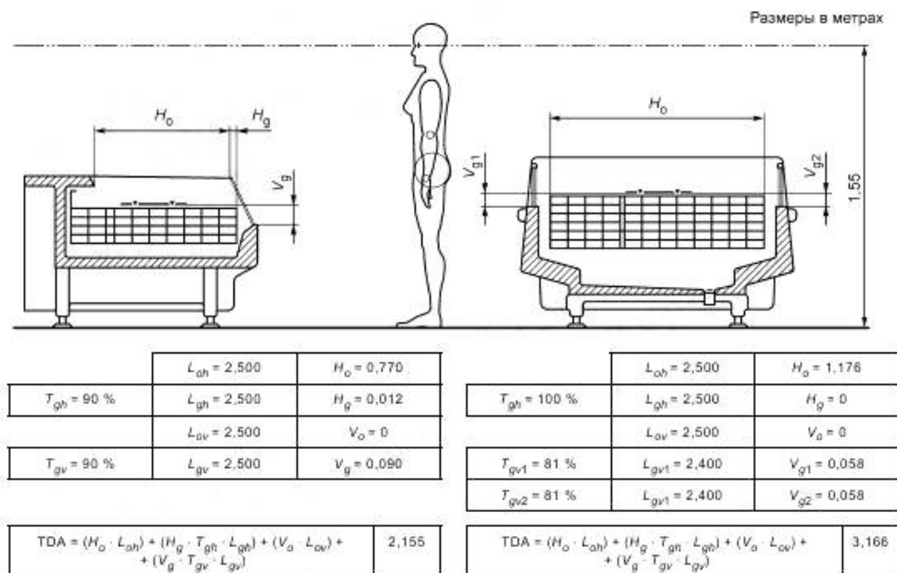
Рисунок А.2 — Горизонтальная открытая витрина островного типа
