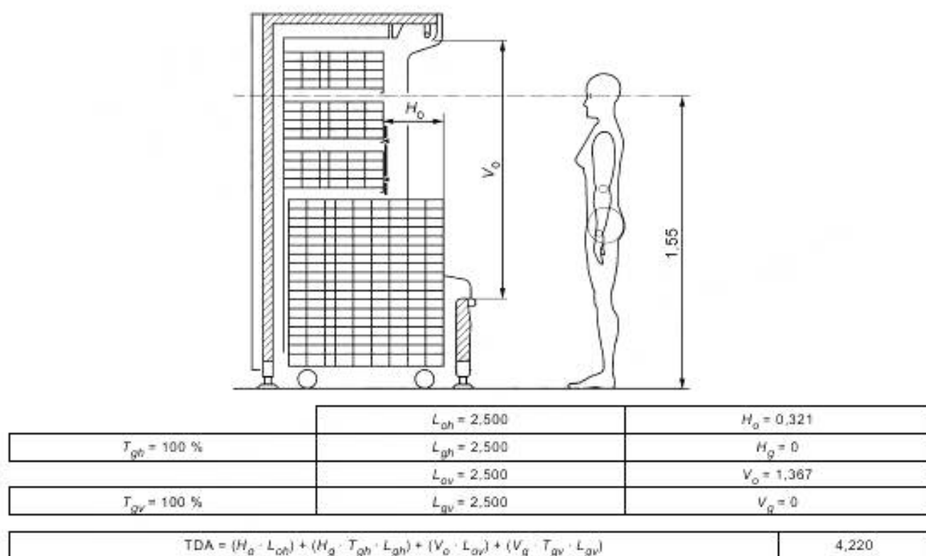
Рисунок А.4 — Вертикальный передвижной шкаф
