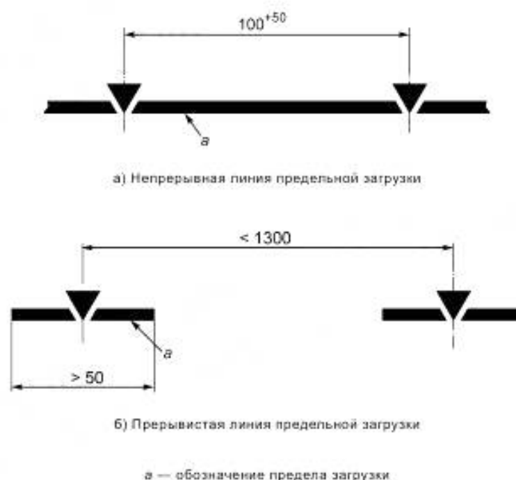
Рисунок 36 — Маркировка предельной загрузки
