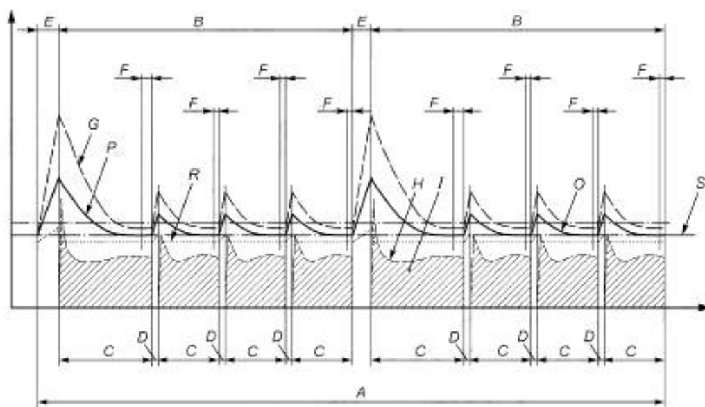
Рисунок 34 — Охлаждение в образце с отводом теплоты из охлаждаемого объема хладагентом. Неустойчивый режим (включение-выключение компрессора)
