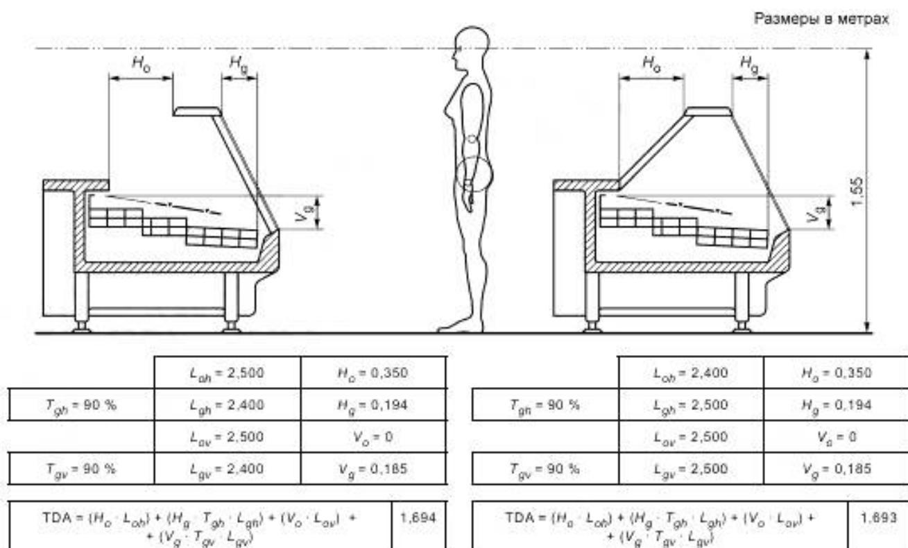
Рисунок А.1 — Горизонтальный открытый прилавок
