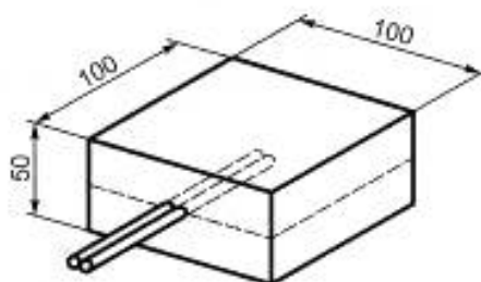
Рисунок 7 — Термометрический контрольный пакет
