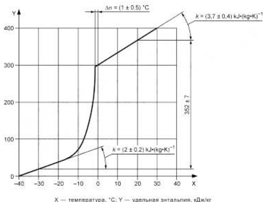
Рисунок 6 — Изменение значения удельной энтальпии наполнителя контрольных пакетов при изменении температуры
