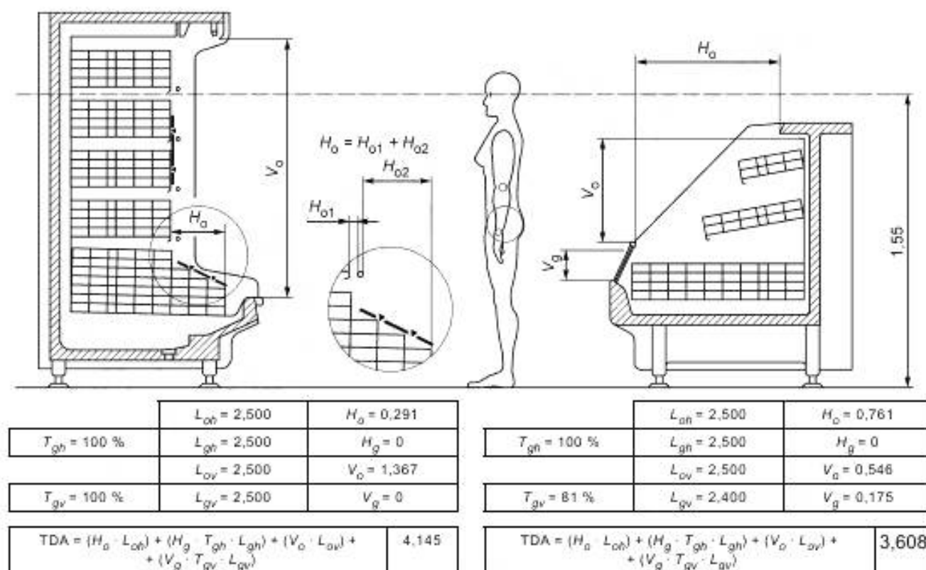
Рисунок А.3 — Вертикальный многоярусный шкаф и горка
