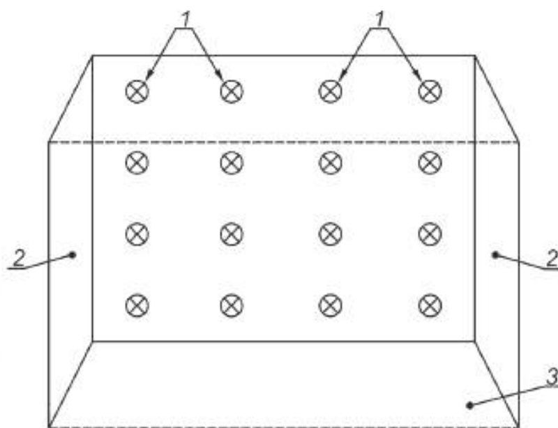
1 – лампы; 2 – алюминиевая фольга; 3 – плоскость образцов
