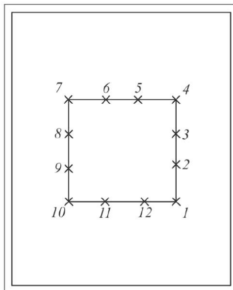
Рисунок 7 – Расположение минимального числа точек ударов молотком
