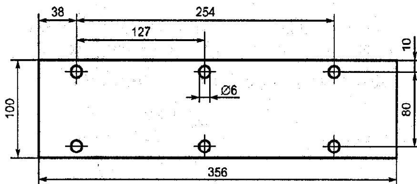
Рисунок 7.22 — Испытуемый образец
