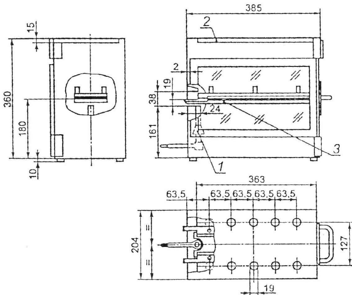
1 — газовая горелка; 2 — вентиляционная щель; 3 — испытуемый образец
