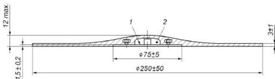
1 — тонкий металлический диск, предназначенный для установки акселерометра и служащий дополнительным центральным элементом жесткости; 2 — углубление для акселерометра (акселерометров).
