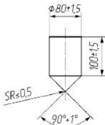
Рисунок G.3 — Испытательный конус
