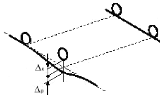
Рисунок 2 – Схема погрешности опорной базы
