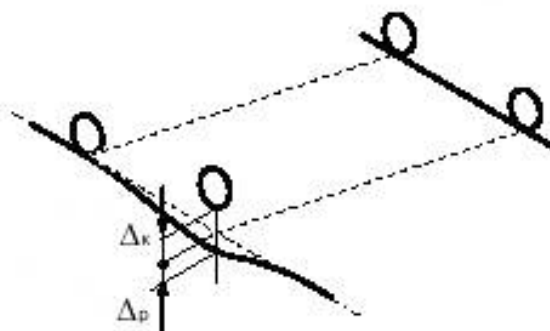
Рисунок 2 – Схема погрешности опорной базы
