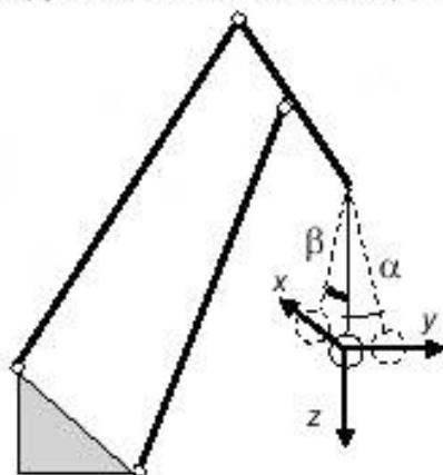
Рисунок 1 – Схема углов отклонения канатов
