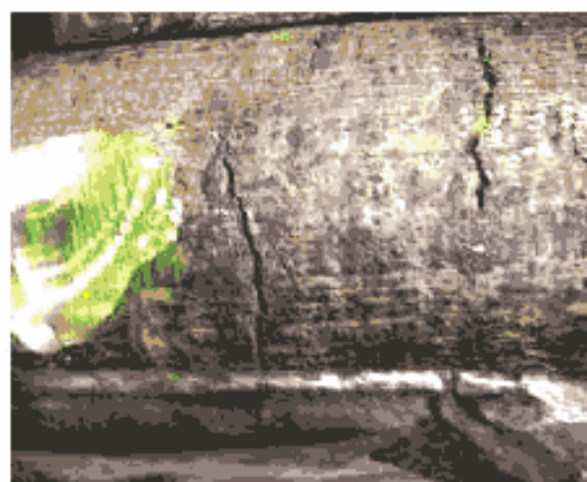
Трещина поперечная на слитке
