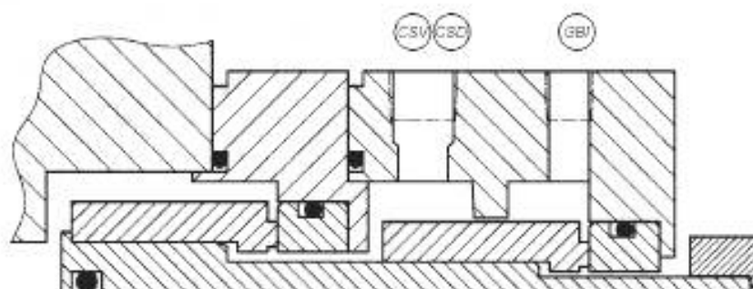
б) 2NC-CS, бесконтактное резервное внутреннее уплотнение
