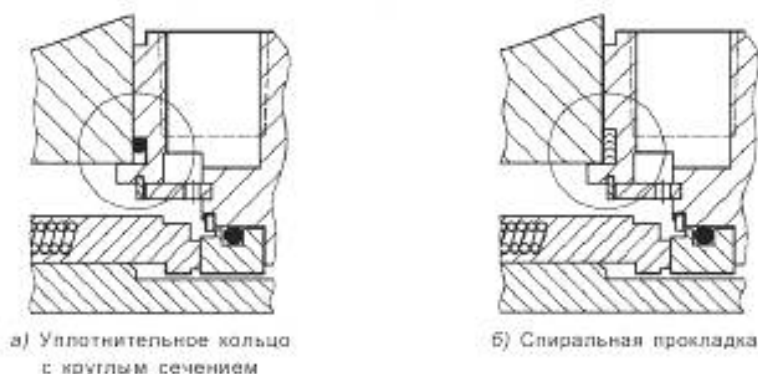
Рисунок 23 — Сопряженные соединения уплотнений
