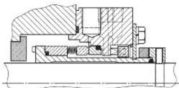
б) Альтернативное (вращающийся узел сифона)
