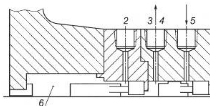
б) Детали камеры уплотнения
