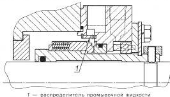
Рисунок 22 — Система распределения промывочной жидкости уплотнения
