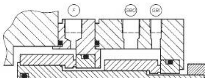
в) конфигурация «двойное уплотнение с подачей буферной жидкости без давления (тандем)», 3NC-FB, бесконтактные уплотнения
