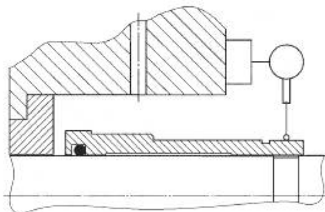
Рисунок 18 — Биение втулки уплотнения
