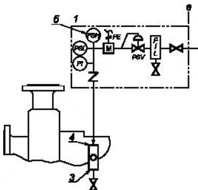
а) Трубопровод и схема измерительного прибора
