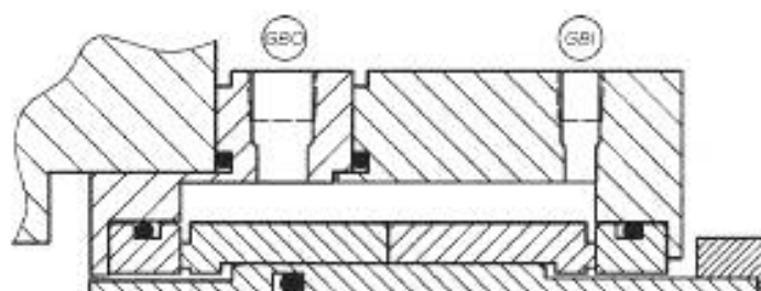
а) Компоновка «спиной к спине», 3NC-BB, бесконтактные уплотнения
