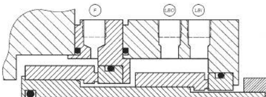
а) 2CW-CW, двойное контактное жидкостное уплотнение
