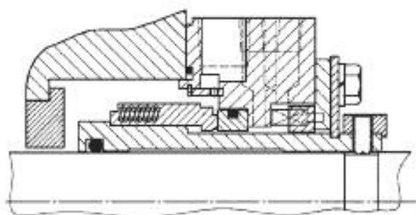
а) Стандартное (вращающийся упругий элемент)
