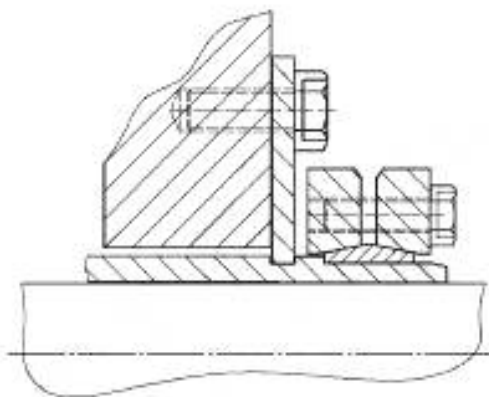
Рисунок 19 — Крепление втулки уплотнения обжимным диском
