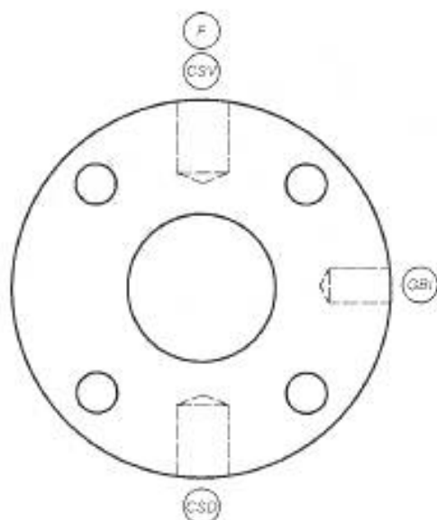
в) Типовая ориентация соединения фланца корпуса для 2CW-CS
