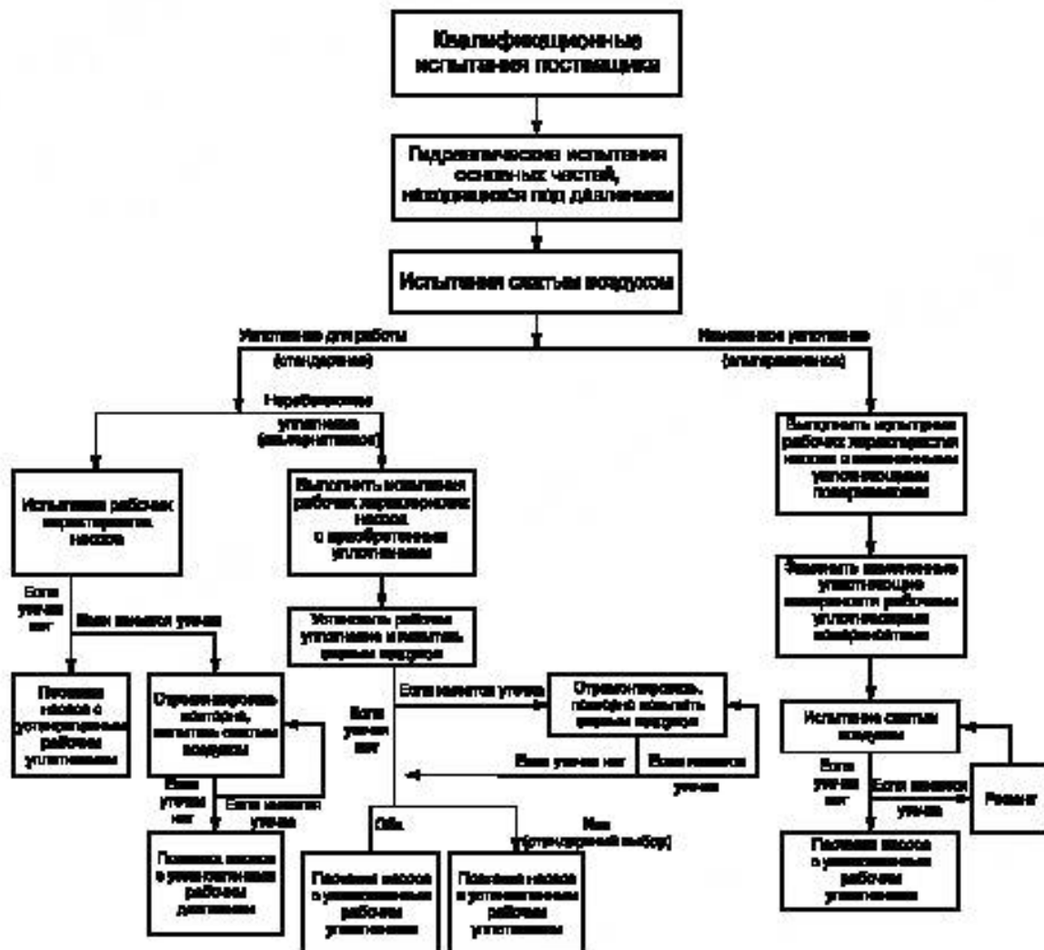
Рисунок 27 — Последовательность действий при проведении испытаний
