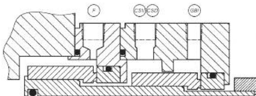
а) 2CW-CS, контактное жидкостное резервное внутреннее уплотнение
