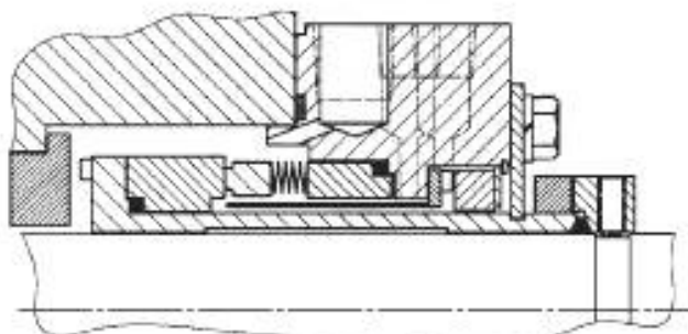
а) Стандартное (неподвижный узел сифона)
