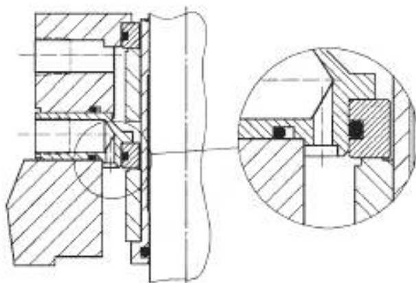
Рисунок 17 — Камера уплотнения/фланец корпуса уплотнения вертикальных насосов
