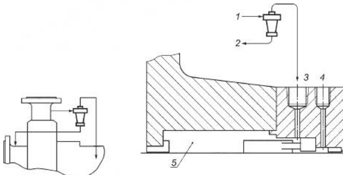
а) Трубопровод и схема измерительного прибора
