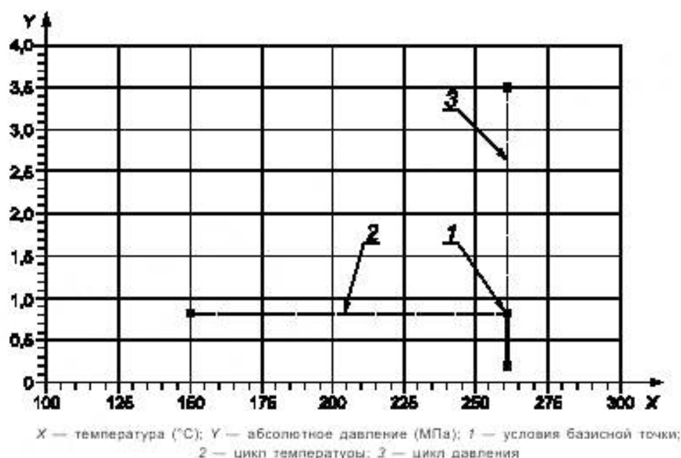
Рисунок 32 — Параметры испытаний минерального масла при воздействии температур от 150 ^{\circ}\text{C} (300 ^{\circ}\text{F} ) до 260 ^{\circ}\text{C} (500 ^{\circ}\text{F} )
