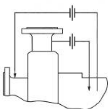
а) Трубопровод и схема измерительного прибора
