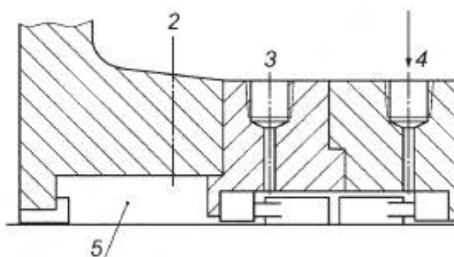
б) Детали камеры уплотнения
