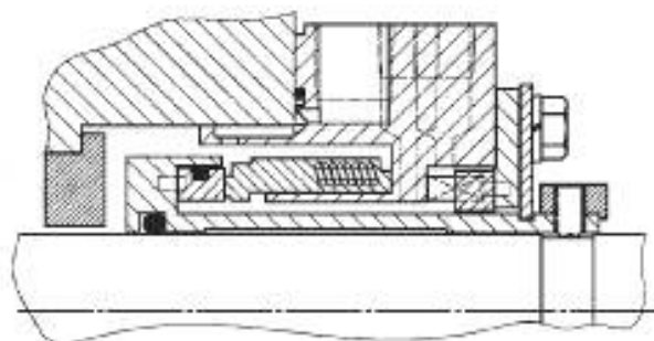
б) Альтернативное (неподвижный упругий элемент)
