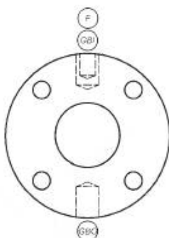
г) Типовая ориентация соединения фланца корпуса
