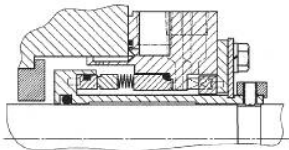
б) Альтернативное (неподвижный узел сифона)
