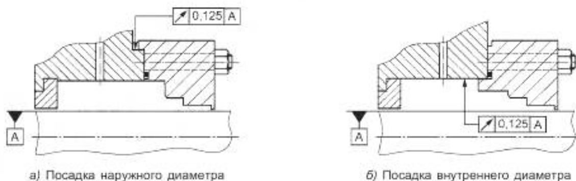
Рисунок 13 — Зарегистрированная соосность камеры уплотнения
