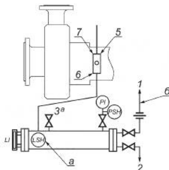
а) Трубопровод и схема измерительного прибора
