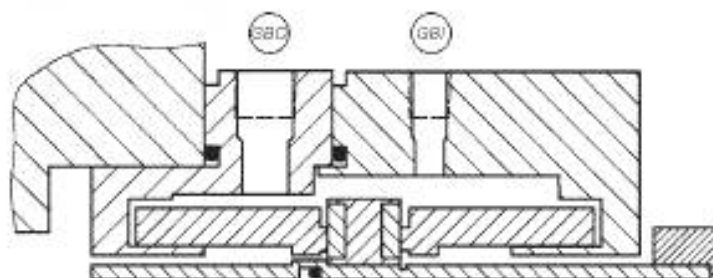
б) конфигурация «двойное уплотнение с подачей барьерной жидкости под давлением («лицом к лицу») 3NC-FF, бесконтактные уплотнения
