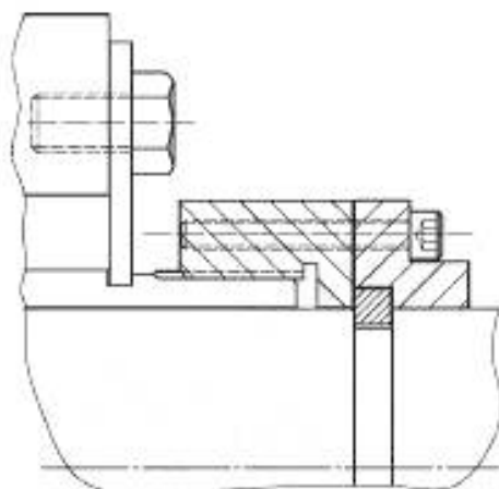
Рисунок 20 — Крепление втулки уплотнения разрезным кольцом
