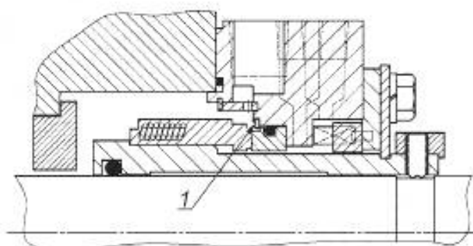
1 — удерживающая деталь (в соответствии с 6.1.1.11)
