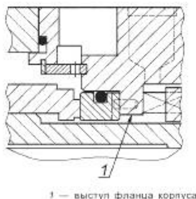
Рисунок 14 — Сечение выступа фланца корпуса
