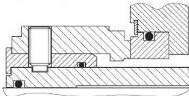
Рисунок 25 — Устройство вспомогательной втулки
