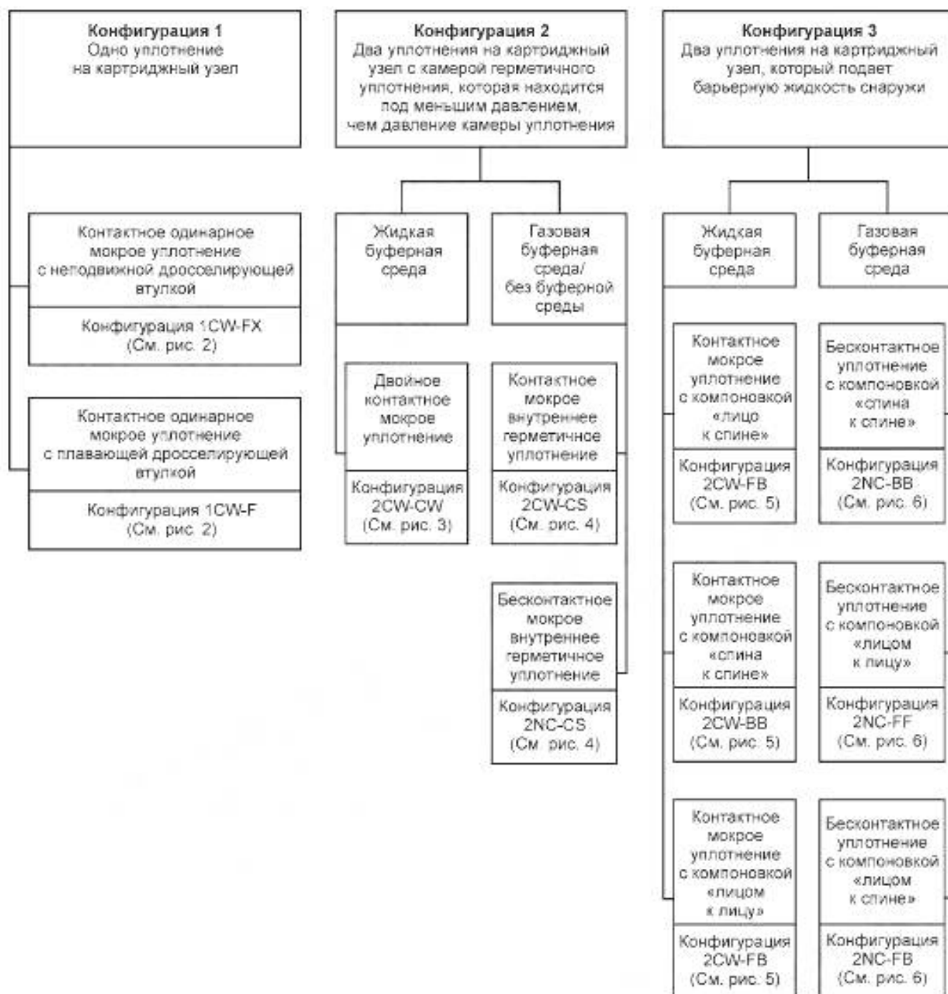
Рисунок 1 — Конфигурация уплотнения
