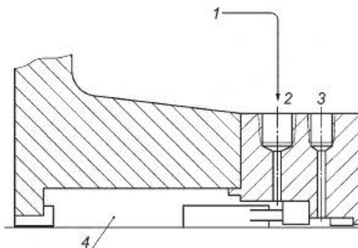
б) Детали камеры уплотнения
