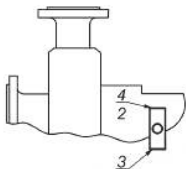
а) Трубопровод и схема измерительного прибора
