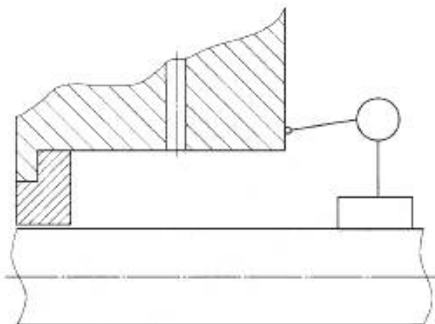
Рисунок 15 — Торцовое биение камеры уплотнения
