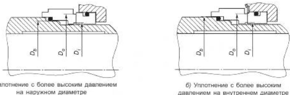
Рисунок 10 — Точки измерений соотношения баланса
