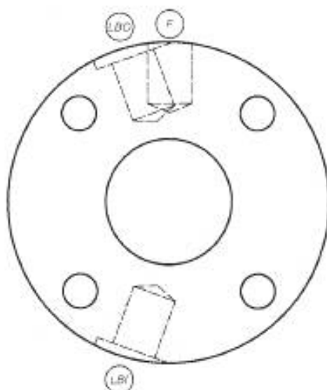
г) Типовая ориентация соединения фланца корпуса
