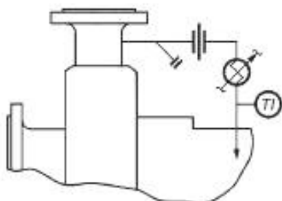
а) Трубопровод и схема измерительного прибора
