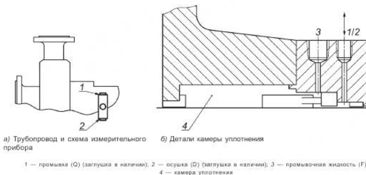
Рисунок Ж.18 — Схема 54 промывки стандартного уплотнения
