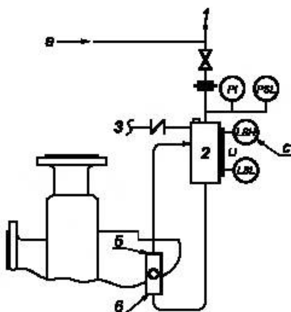
а) Трубопровод и схема измерительного прибора
