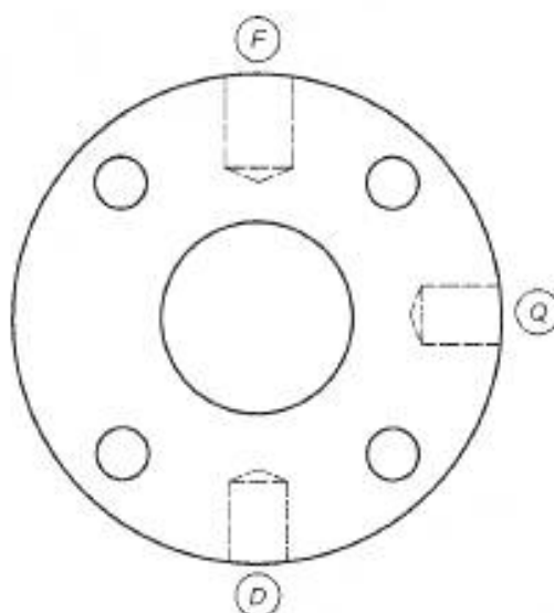
в) Типовая ориентация соединения фланца корпуса
