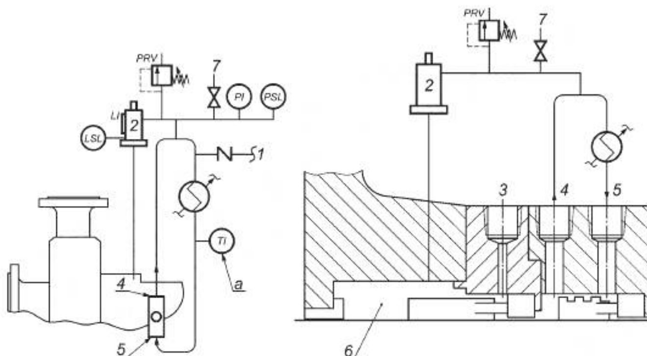
а) Трубопровод и схема измерительного прибора
