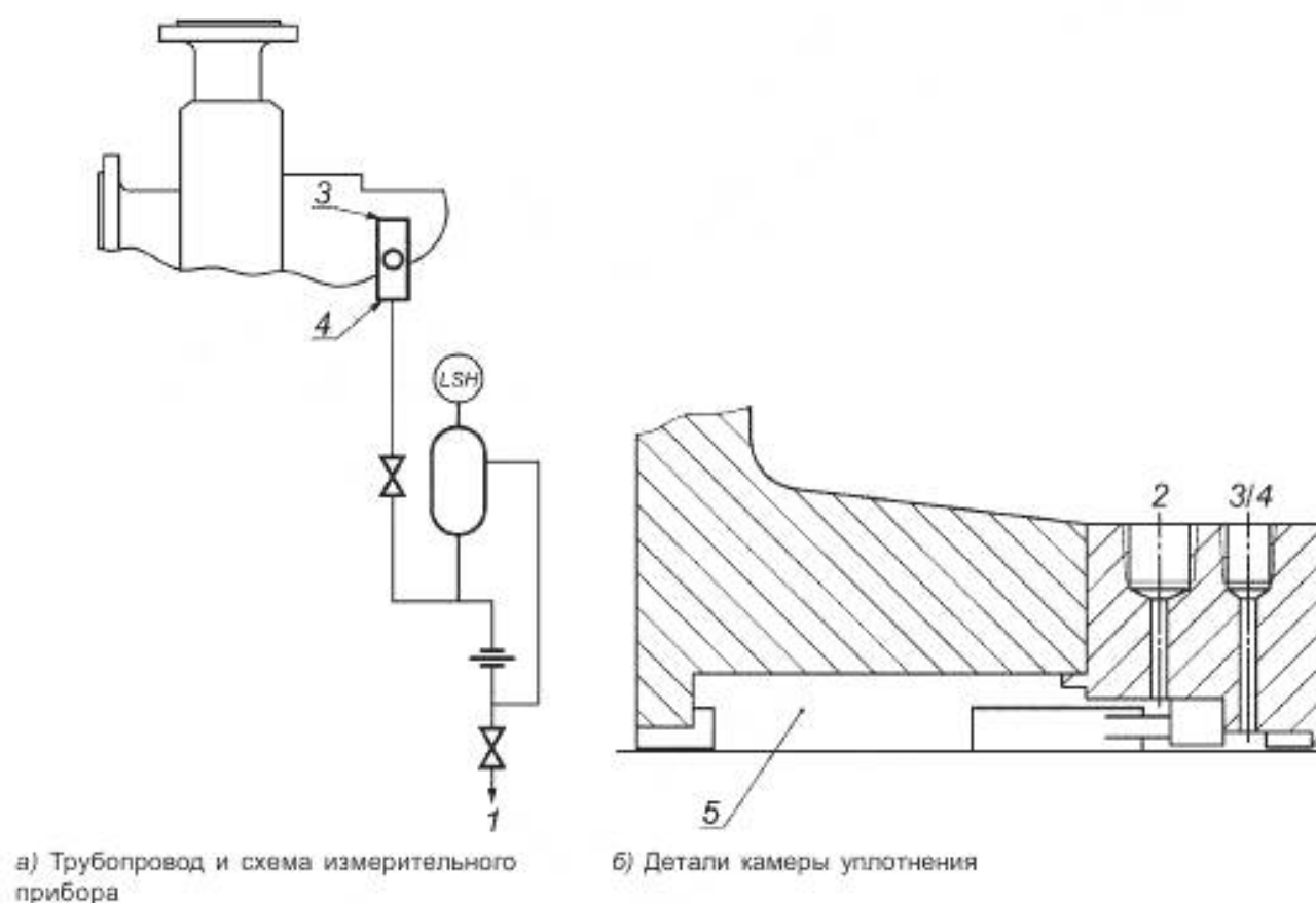
Рисунок Ж.20 — Схема промывки 62 стандартного уплотнения
