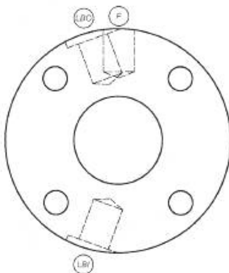
б) Типовая ориентация соединения фланца корпуса
