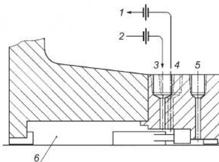
б) Детали камеры уплотнения
