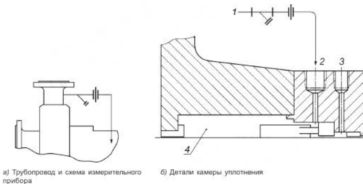
Рисунок Ж.3 — Схема промывки 11 стандартного уплотнения
