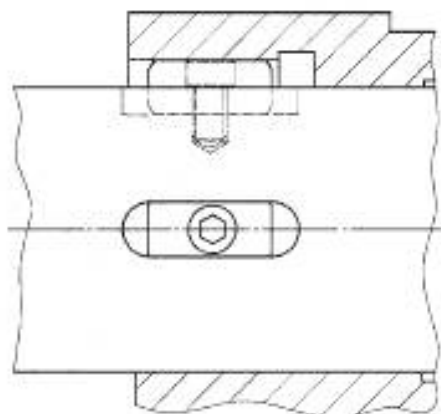
Рисунок 24 — Крепление шпонки к валу
