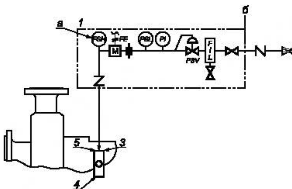
а) Трубопровод и схема измерительного прибора
