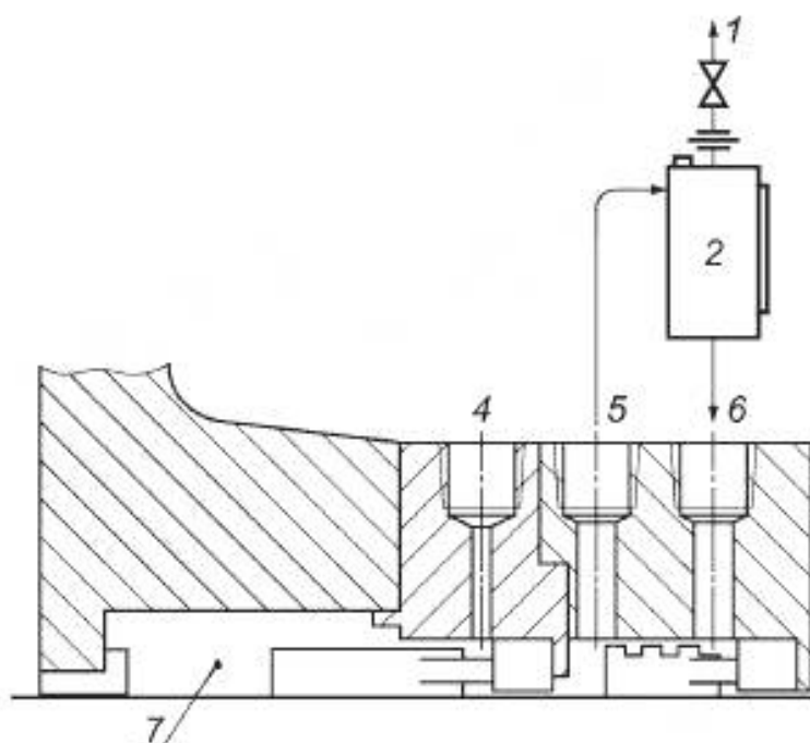
б) Детали камеры уплотнения
