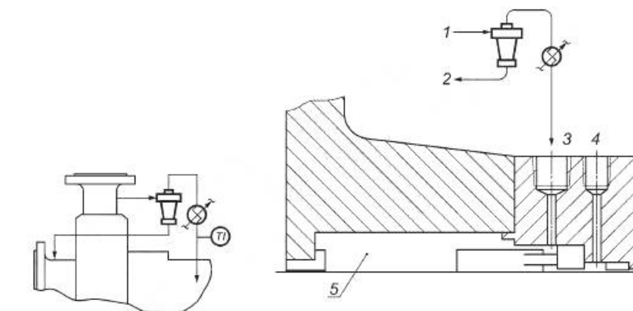
а) Трубопровод и схема измерительного прибора
