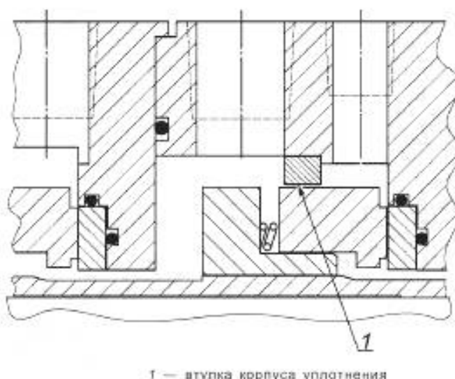
1 — втулка корпуса уплотнения
