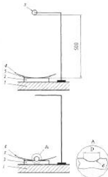
1 – неподвижный стол; 2 – испытуемый образец; 3 – лицевая сторона плиты; 4 – копировальная бумага; 5 – стальной шарик; 6 – цветной отпечаток
