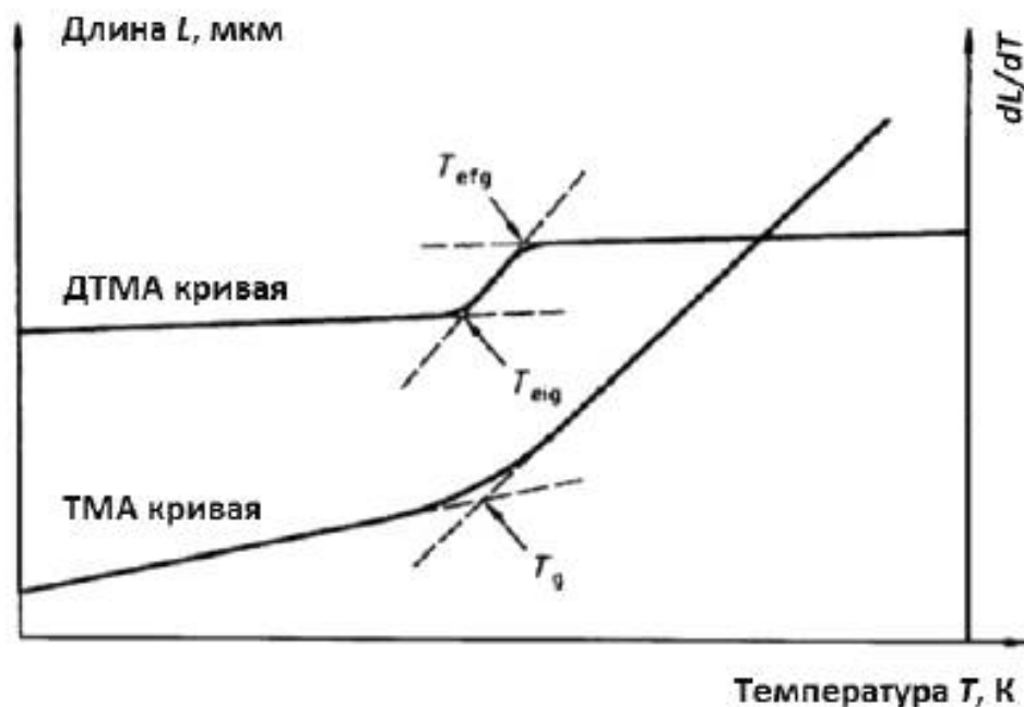
Рисунок 3 – Определение температуры стеклования
