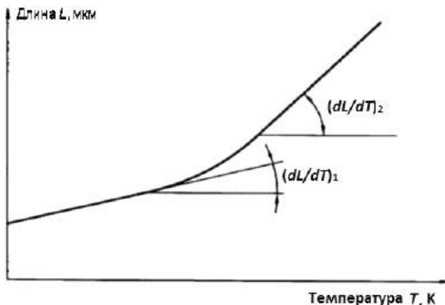
Рисунок 1 – Определение коэффициента линейного теплового расширения
