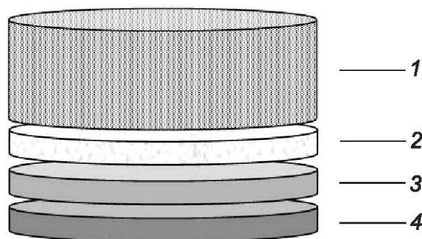
1 — вспененный полиэтилен (EPE); 2 — белый картон (PAP); 3 — оловянная фольга (Tin); 4 — поливинилиденхлорид (PVDC)
