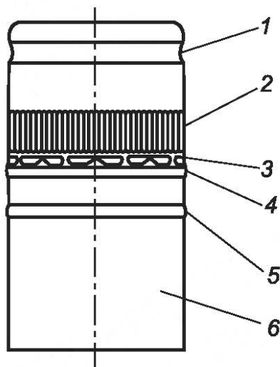
1 — закругленный бортик, удерживающий уплотнительную прокладку (вкладыш); 2 — накатка (гофрировка); 3 — перемычки (мостики); 4 — линия защиты (при первом вскрытии у колпачка появляются нарушения его целостности, что гарантирует защиту от фальсификации); 5 — опорная часть; 6 — нижняя часть корпуса («юбка»)
