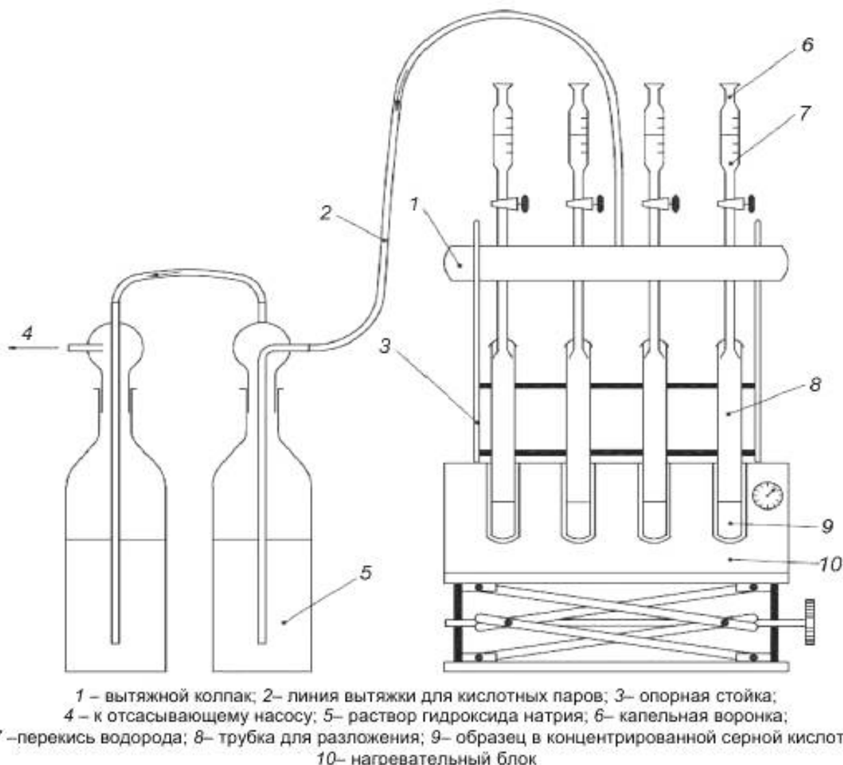
Рисунок А.1 — Аппаратура для метода В. Химическое разложение
