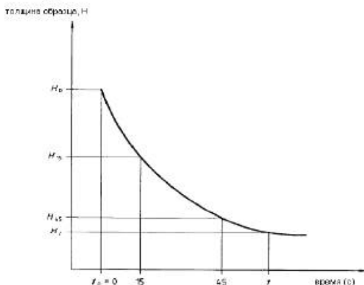
Рисунок 5 — Стандартная кривая текучести, определенная методом 1
