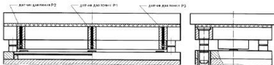
Рисунок 4 – Испытательная форма с датчиками
