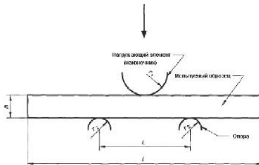
Рисунок 2 — Конфигурация нагружения
