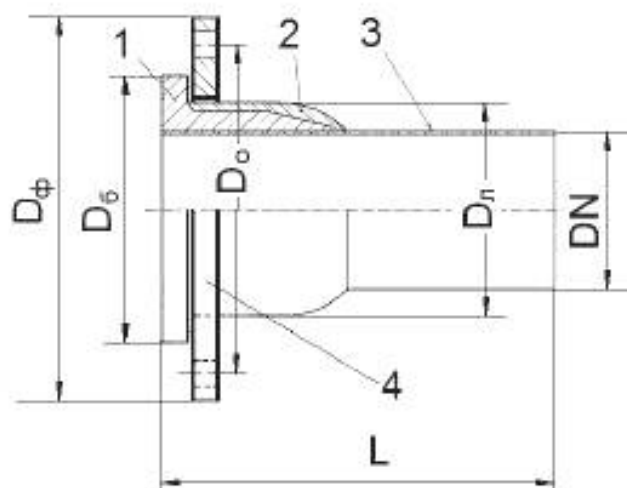
Рисунок А.8 – Фиксированный фланец
