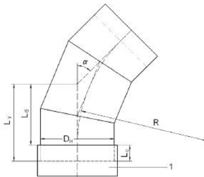
1 – муфта; D_H – наружный диаметр трубы; L_y – уложенная длина отвода; L_6 – базовая длина; L_0 – длина соединения; \alpha – угол отвода; R – радиус отвода.
