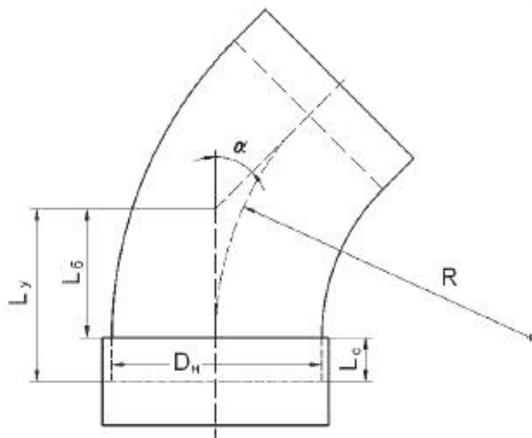
Рисунок А.3 Сплошной отвод
