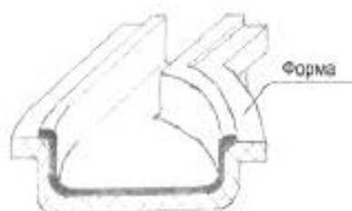
Рисунок А.1 – Формовой способ изготовления корпуса вентилятора
