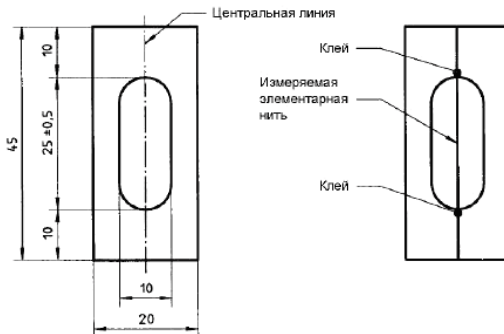
Рисунок 1 – Рамка для крепления элементарной нити
