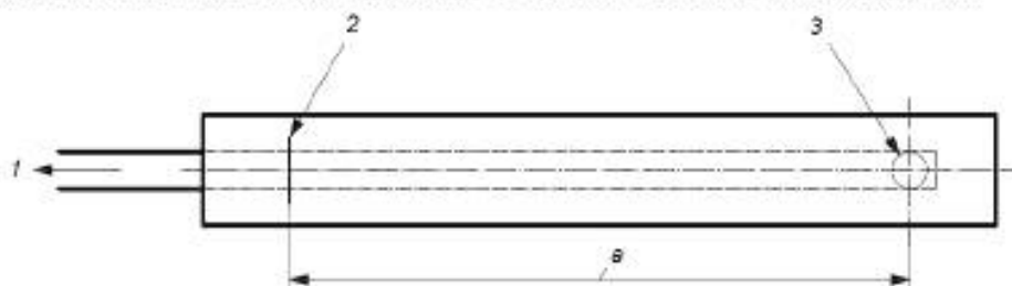
1 – натяжение; 2 – лезвие резака; 3 – направляющий стержень; a \leq 2,50 м Рисунок А.1 – Оборудование для нарезания испытуемых проб длиной до 5 м
