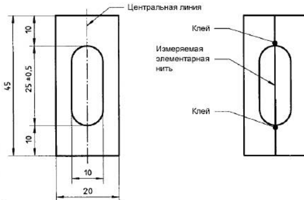
Рисунок 1 – Рамка для крепления элементарной нити
