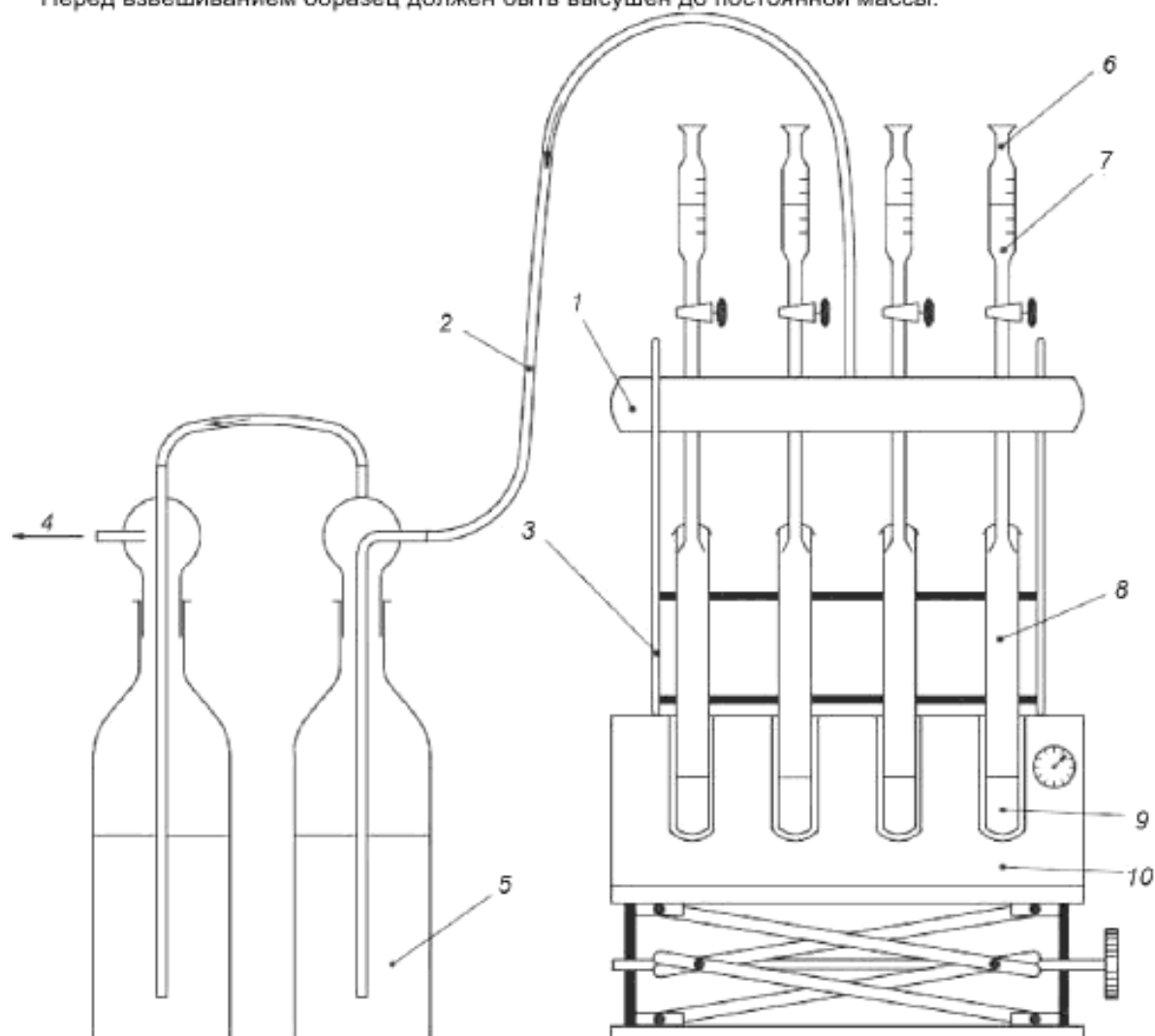
1 – вытяжной колпак; 2– линия вытяжки для кислотных паров; 3– опорная стойка; 4 – к отсасывающему насосу; 5– раствор гидроксида натрия; 6– капельная воронка; 7 –перекись водорода; 8– трубка для разложения; 9 – образец в концентрированной серной кислоте; 10– нагревательный блок
