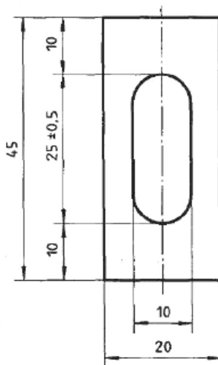
Рисунок 1 – Рамка для крепления образца
