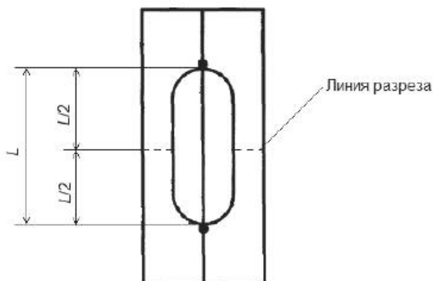
Рисунок 3 – Разрез рамки для крепления
