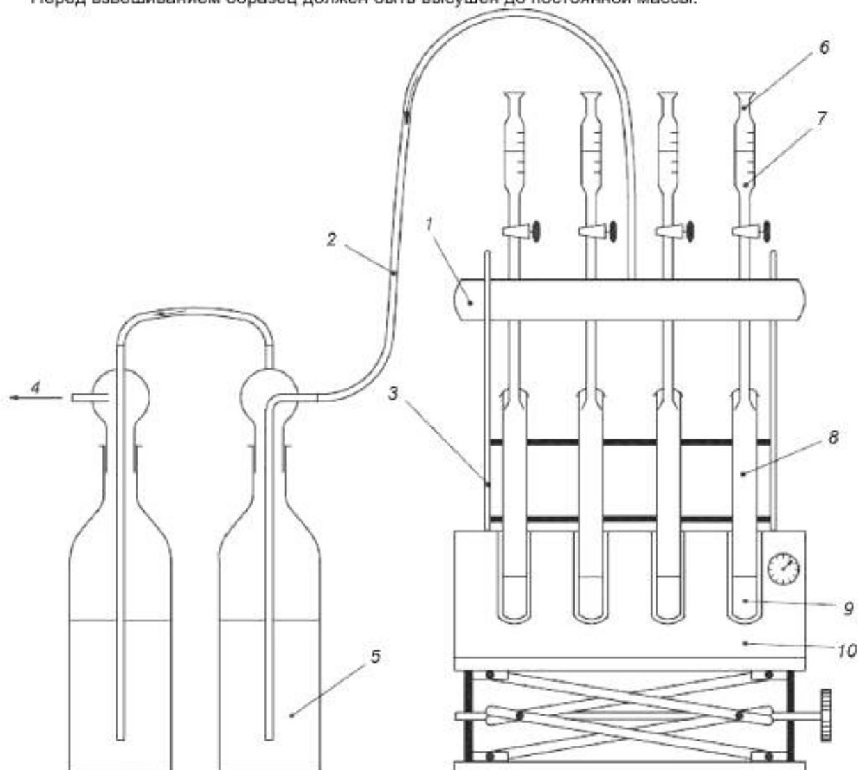
1 – вытяжной колпак; 2 – линия вытяжки для кислотных паров; 3 – опорная стойка; 4 – к отсасывающему насосу; 5 – раствор гидроокиси натрия; 6 – каплевальная воронка; 7 – перекись водорода; 8 – трубка для разложения; 9 – образец в концентрированной серной кислоте; 10 – нагревательный блок
