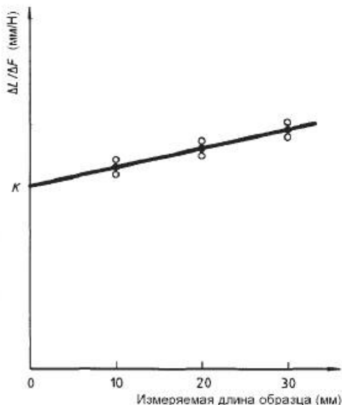
Рисунок А.1 — Определение податливости системы K
