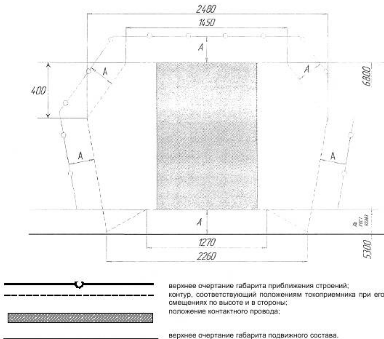
Рисунок 1 — Расстояния между сооружениями, устройствами контактной сети, токоприемниками и подвижным составом
