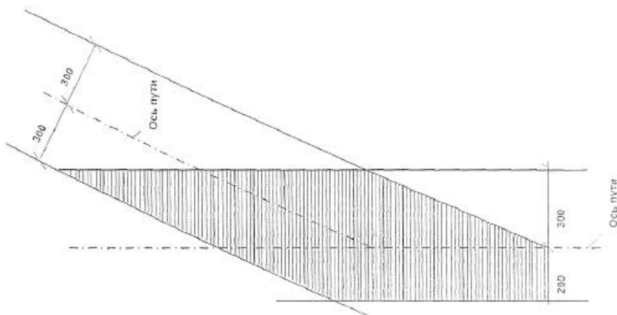
Рисунок 2 — Расположение на плоскости пути обыкновенного стрелочного перевода проекции точки пересечения контактных проводов воздушной стрелки
