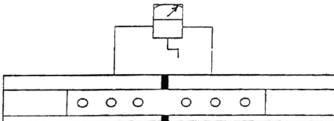
Рисунок 1 – Общая схема измерения электрического сопротивления изолирующего стыка
