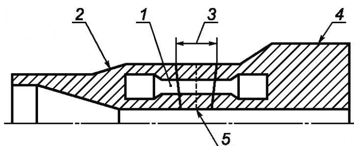
а — Расположение образца для испытания на растяжение
