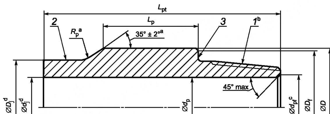
Рисунок В.11 — Искусственный дефект (надрез) для неразрушающего контроля тел труб
