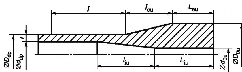
с — Наружная высадка, группы прочности X , G , S (все размеры) и группы прочности D , E (бурильные трубы наружным диаметром тела трубы 88,90 мм и толщиной стенки 9,35 мм)
