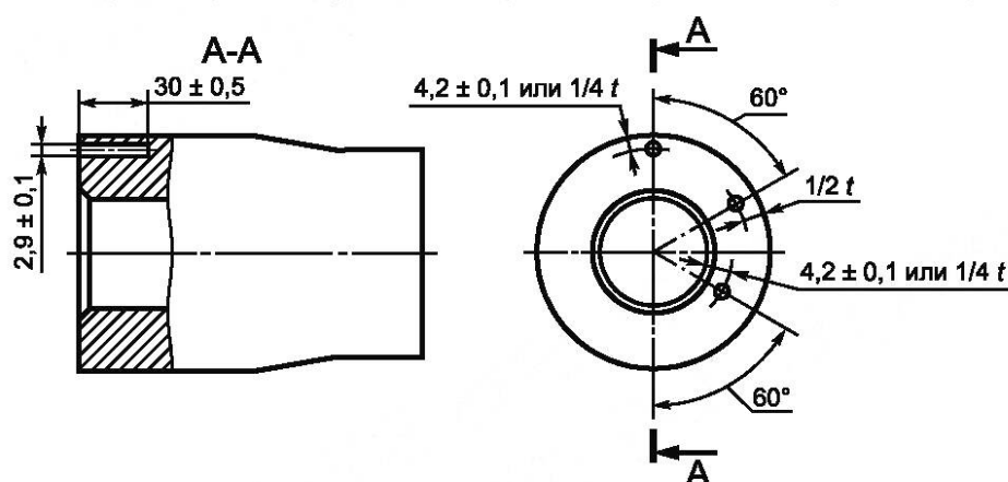
t — толщина стенки тела трубы
