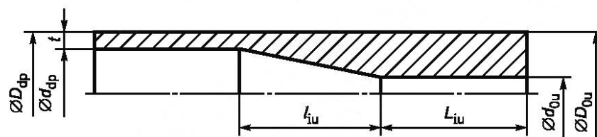
а — Внутренняя высадка, все группы прочности
