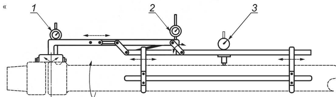
е — Измерение угловой и параллельной несоосности тела буровой трубы и замка 1 — угловая несоосность; 2 — параллельная несоосность; 3 — прямолинейность трубы».
