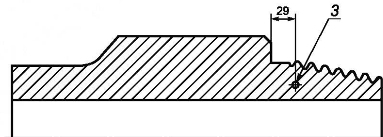
b — Участок контроля твердости ниппеля (при необходимости)
