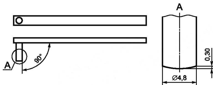
А — Скругленный контактный наконечник
