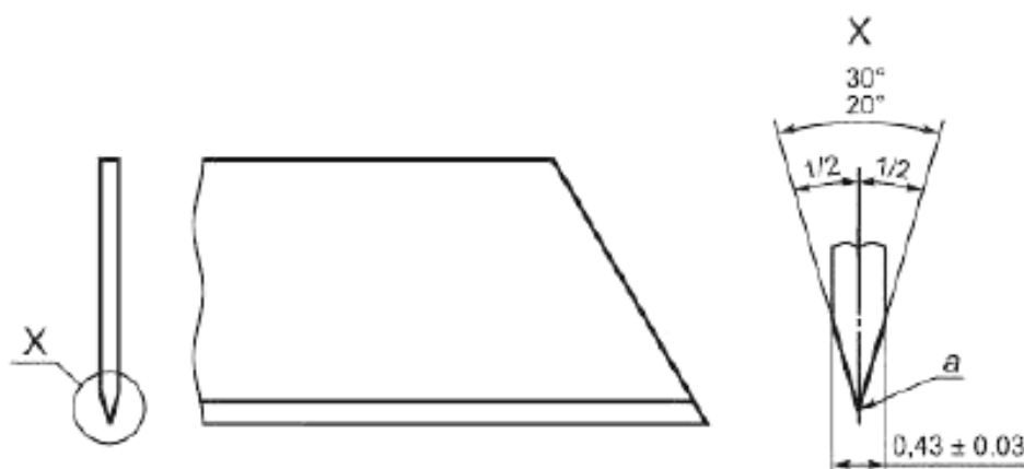
1 – режущие кромки; а – направление разреза
