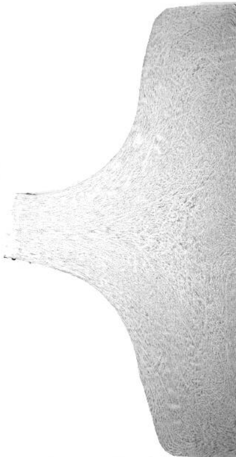
Рисунок А.3 – Эталон № 3 (однородная макроструктура ступицы колеса и центра)
