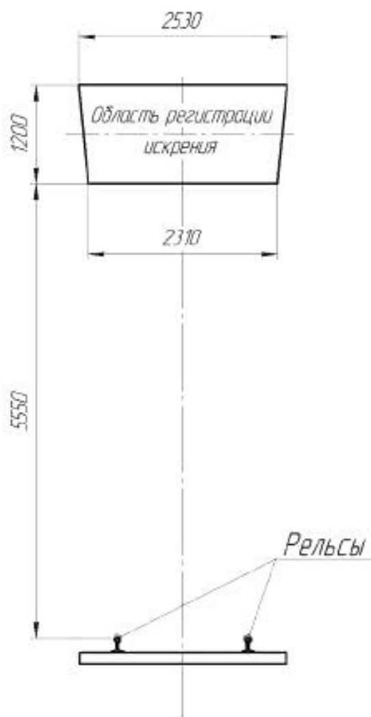
Рисунок 3 — Размеры и положение области регистрации искрения
