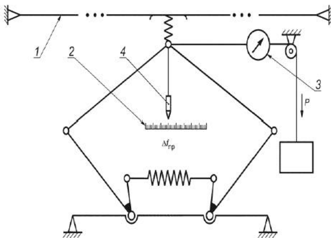
1 — контактный провод; 2 — измерительная линейка; 3 — динамометр; 4 — отвес
