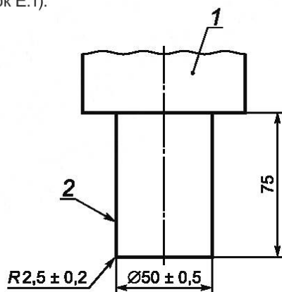
Рисунок Е.1 — Плунжер
