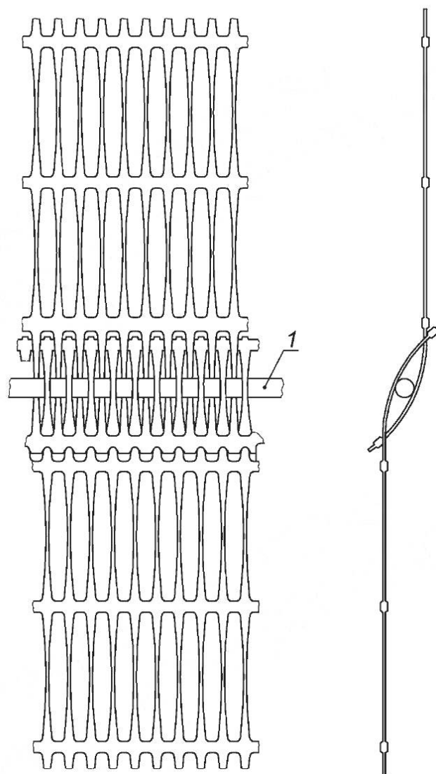
1 — канвовая игла
