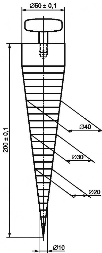
Рисунок Л.5 — Пример измерительного конуса
