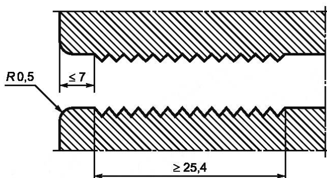
Рисунок Л.2 — Пример деталей зубчатых поверхностей
