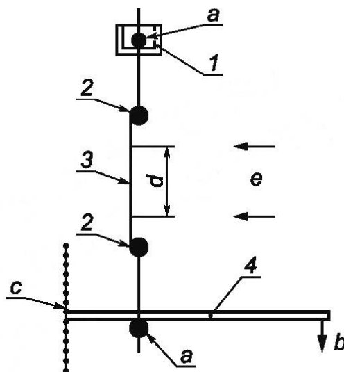
1 — жесткая рамка; 2 — зажим для испытуемого образца; 3 — испытуемый образец; 4 — грузоподъемник; а — сферическая насадка; b — нагрузка; с — регулируемый центр вращения для постоянной нагрузки; d — номинальная длина; e — удаленное измерение с помощью экстензометра
