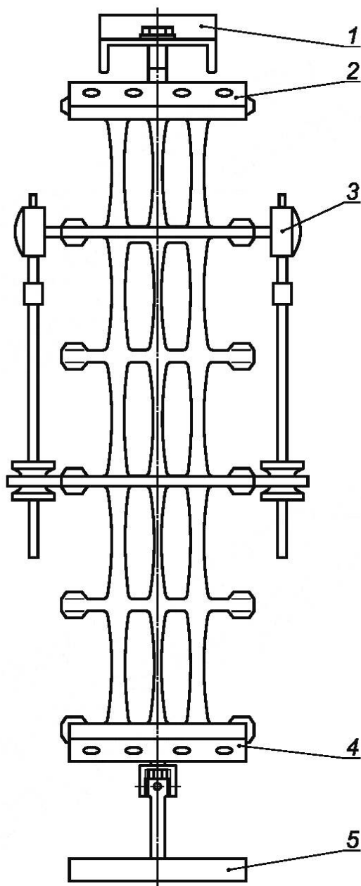
Рисунок К.3 — Испытательная установка для проверки прочности
