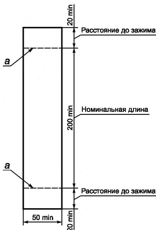
Рисунок К.1 — Детали образца для испытания
