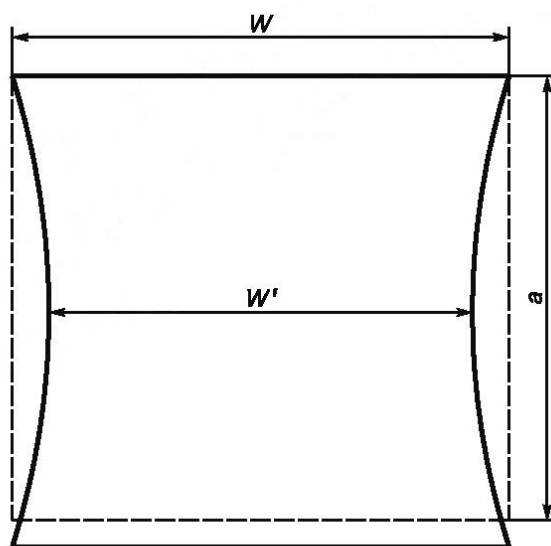
Рисунок К.2 — Размер сжатия образца
