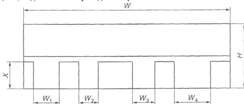
Рисунок 6 – Определение площади нахлеста для многослойной черепицы
