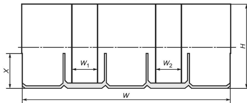
Рисунок 9 — Определение площади нахлеста слоев (второго слоя третьим) в видимой части трехслойной черепицы».
