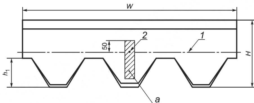
б) Двухслойная черепица
