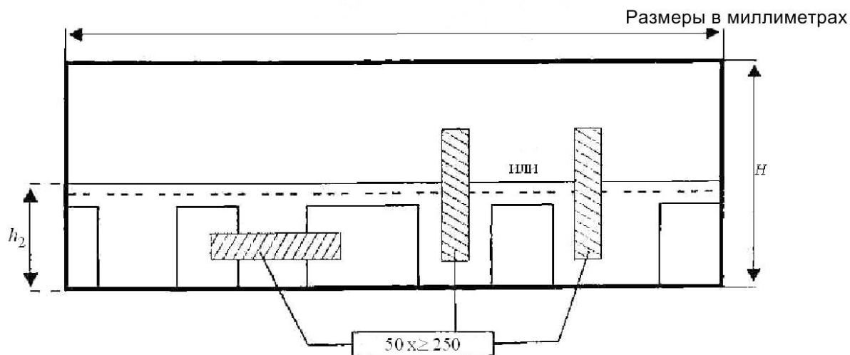
Рисунок 2 – Пример вырубki образцов из многослойной черепицы для определения максимальной силы растяжения
