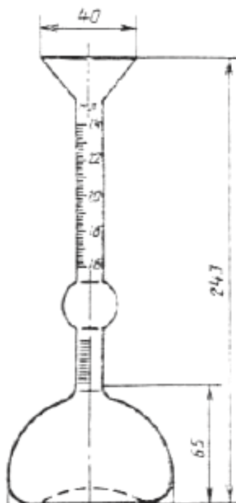
Рисунок 1 — Прибор Ле-Шателье
