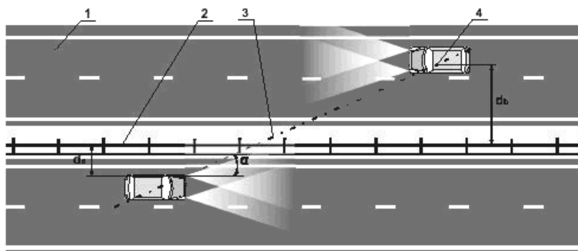
1 – проезжая часть; 2 – ось экрана; 3 – луч света; 4 – положение глаз водителя; d_0 – расстояние от глаз водителя до противоослепляющего экрана; d_b – расстояние от фары транспортного средства, являющегося источником луча падающего света, до противоослепляющего экрана Рисунок Б.2 – Схема расположения транспортных средств в горизонтальной плоскости
