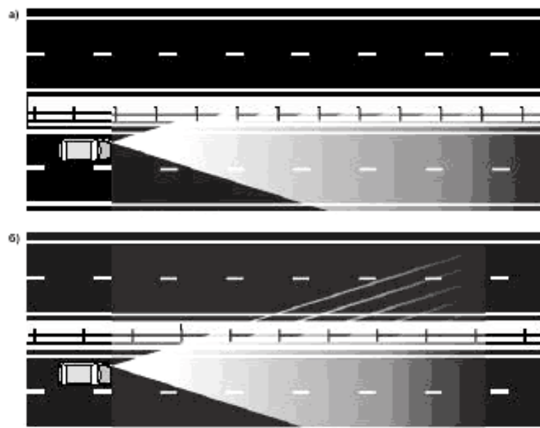
Рисунок 1 – Схема задерживания экраном светового потока а) – полное задерживание светового потока; б) – частичное задерживание светового потока
