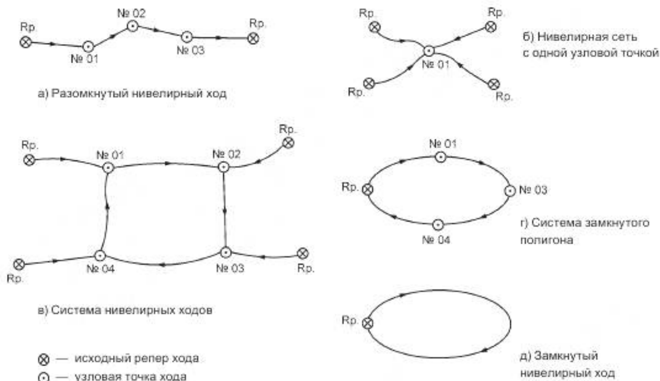
Рисунок 1 — Виды нивелирного хода
