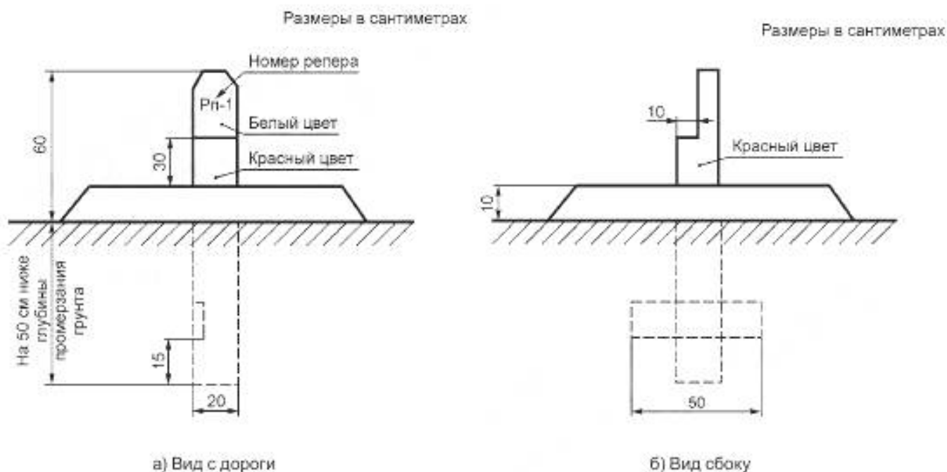
Рисунок Г.1 — Закладка реперов долговременного закрепления
