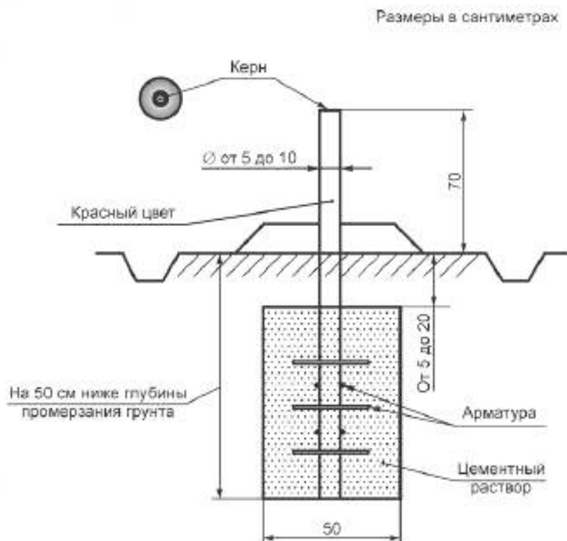
Рисунок Г.2 — Закладка геодезических пунктов долговременного закрепления
