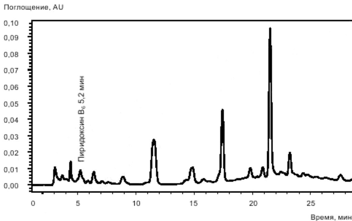
Рисунок В.6 – Хроматограмма нектара из яблок, черноплодной рябины и малины, обогащенного витаминами и минеральными веществами с хроматографическим пиком витамина B 6
