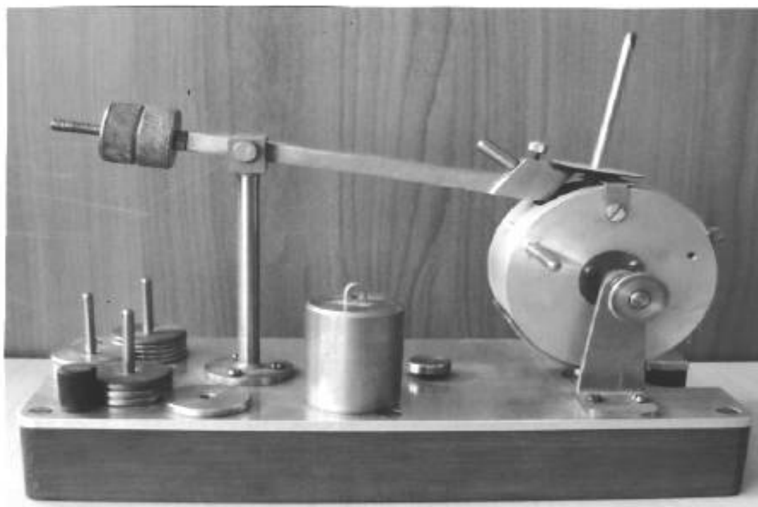
Рисунок 2 – Прибор для определения чувствительности спичек к воспламенению
