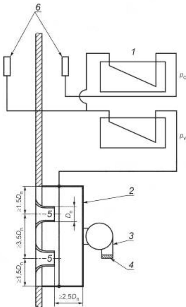
1 — манометры давления; 2 — разгрузочная камера; 3 — вытяжной вентилятор; 4 — заслонка; 5 — сопло; 6 — трубка забора; D_n — диаметр горловины сопла, м; p_c — давление выравнивания в отсеке; p_v — скоростной напор через сопло
