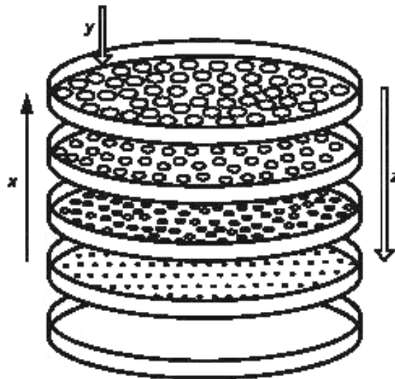
Рисунок 1 — Схема устройства для ситового анализа
