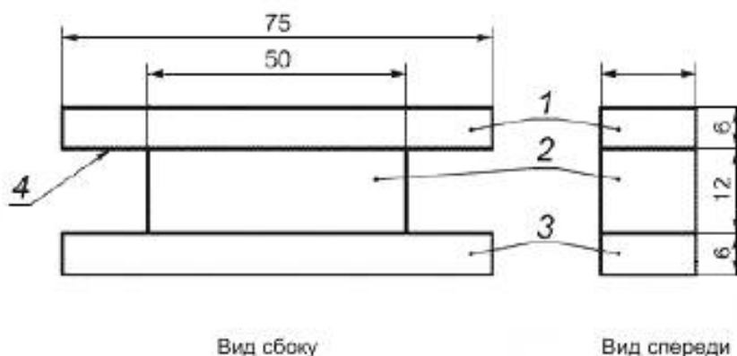
Рисунок А.1 — Испытываемый образец
