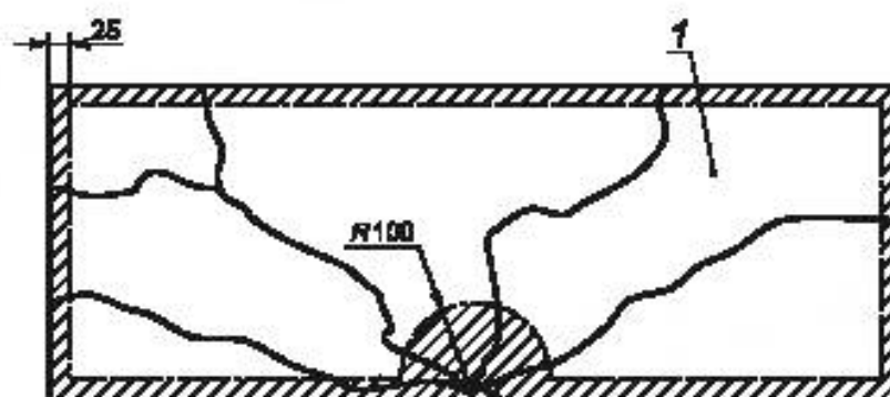
1 — области, образующиеся при разрушении термоупрочненного стекла
