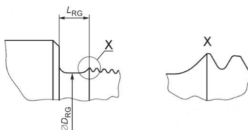
Рисунок 12 — Разгрузочная канавка
