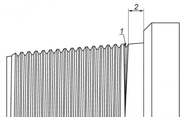
1 — конечная резьба на полную глубину; 2 — длина основания штифта
