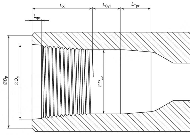
Рисунок 13 — Проточка муфты
