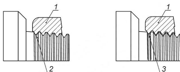
1 — профильный калибр; 2 — резьба на полную глубину; 3 — резьба на неполную глубину
