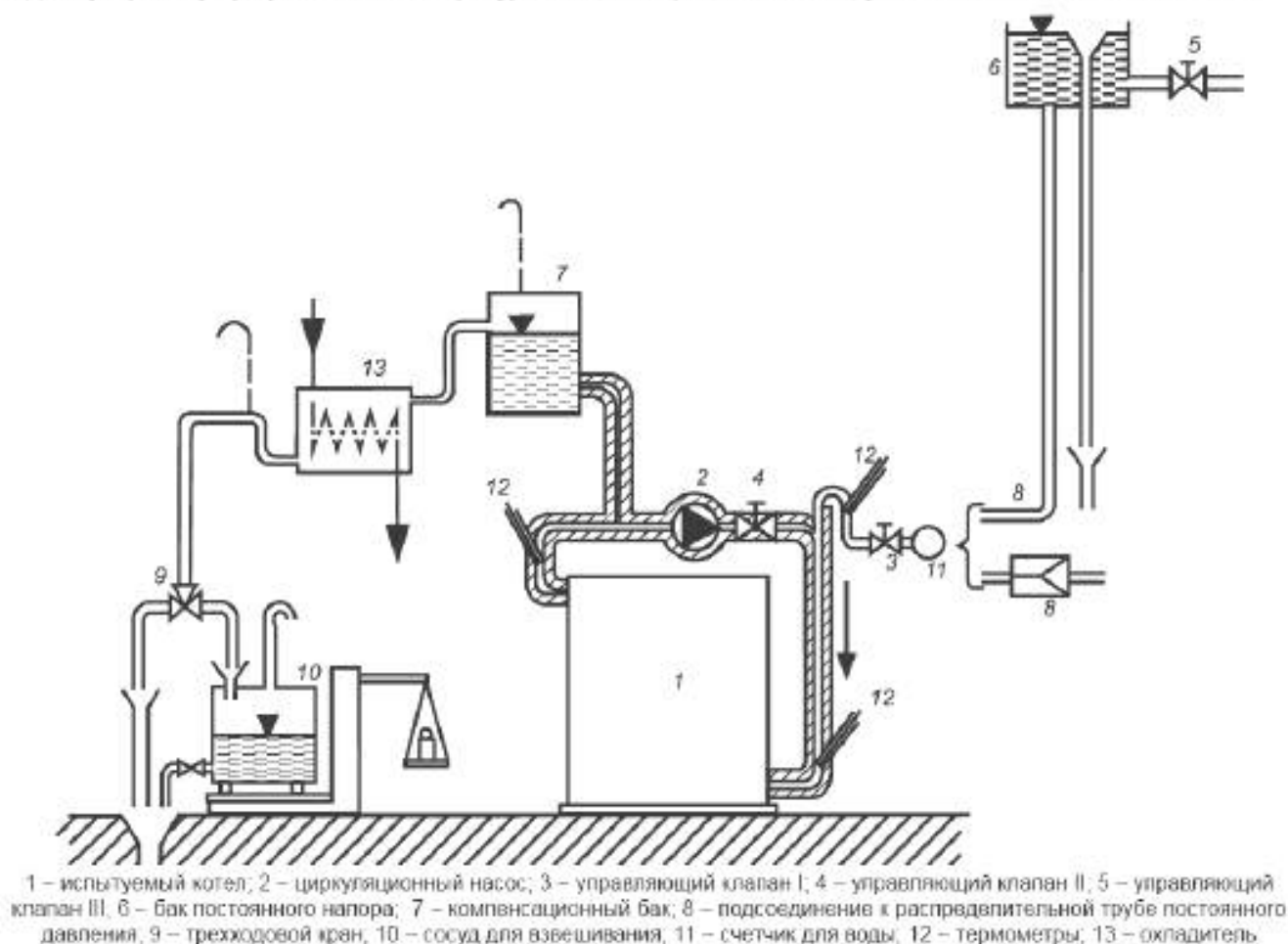
Рисунок 1 — Испытательный стенд с прямой циркуляцией
