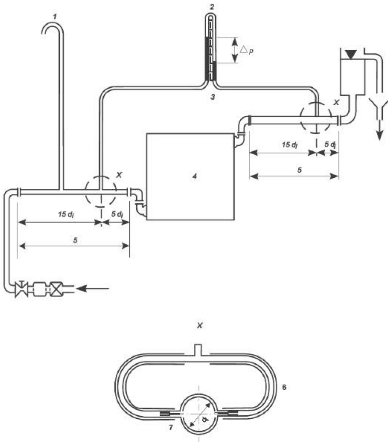
Рисунок 3 – Устройство для определения гидравлического сопротивления
