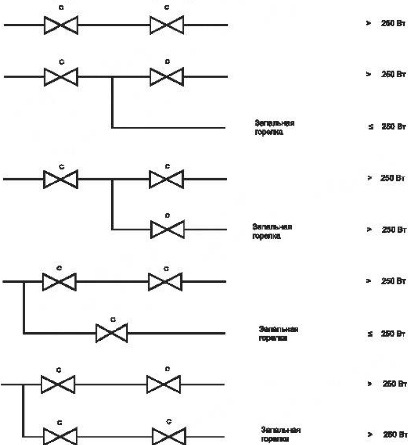
Рисунок Н.5 — Подводимая тепловая мощность до 70 кВт
