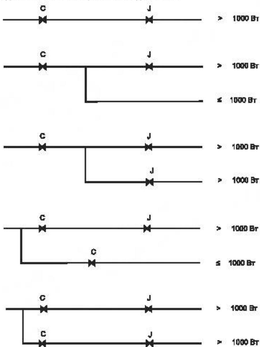
Рисунок Н.2 — Подводимая тепловая мощность до 150 кВт
