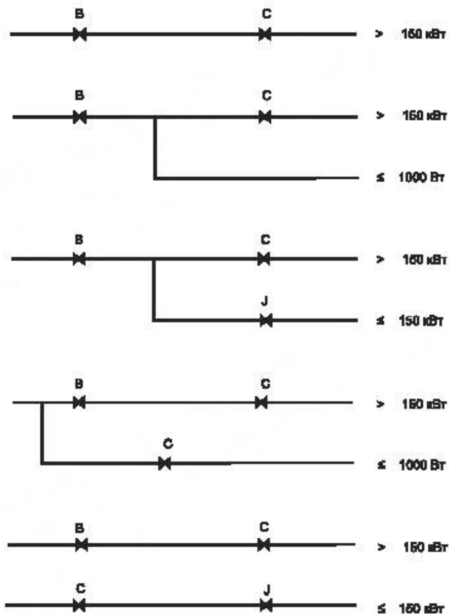
Рисунок Н.3 — Подводимая тепловая мощность до 300 кВт
