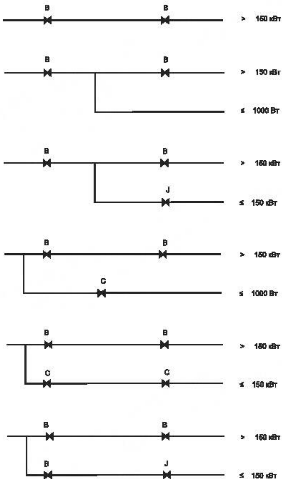
Рисунок Н.7 — Подводимая тепловая мощность до 300 кВт
