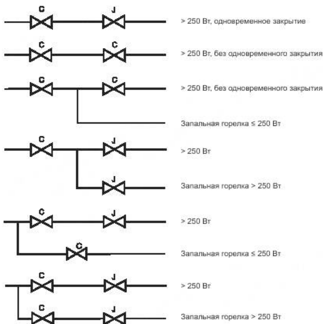
Рисунок Н.1 — Подводимая тепловая мощность до 70 кВт
