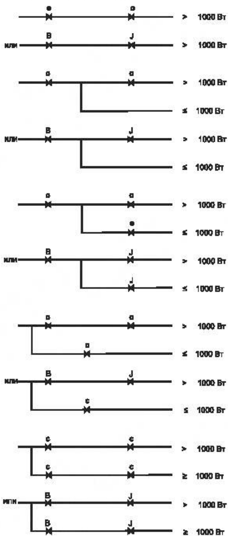
Рисунок Н.6 — Подводимая тепловая мощность до 150 кВт
