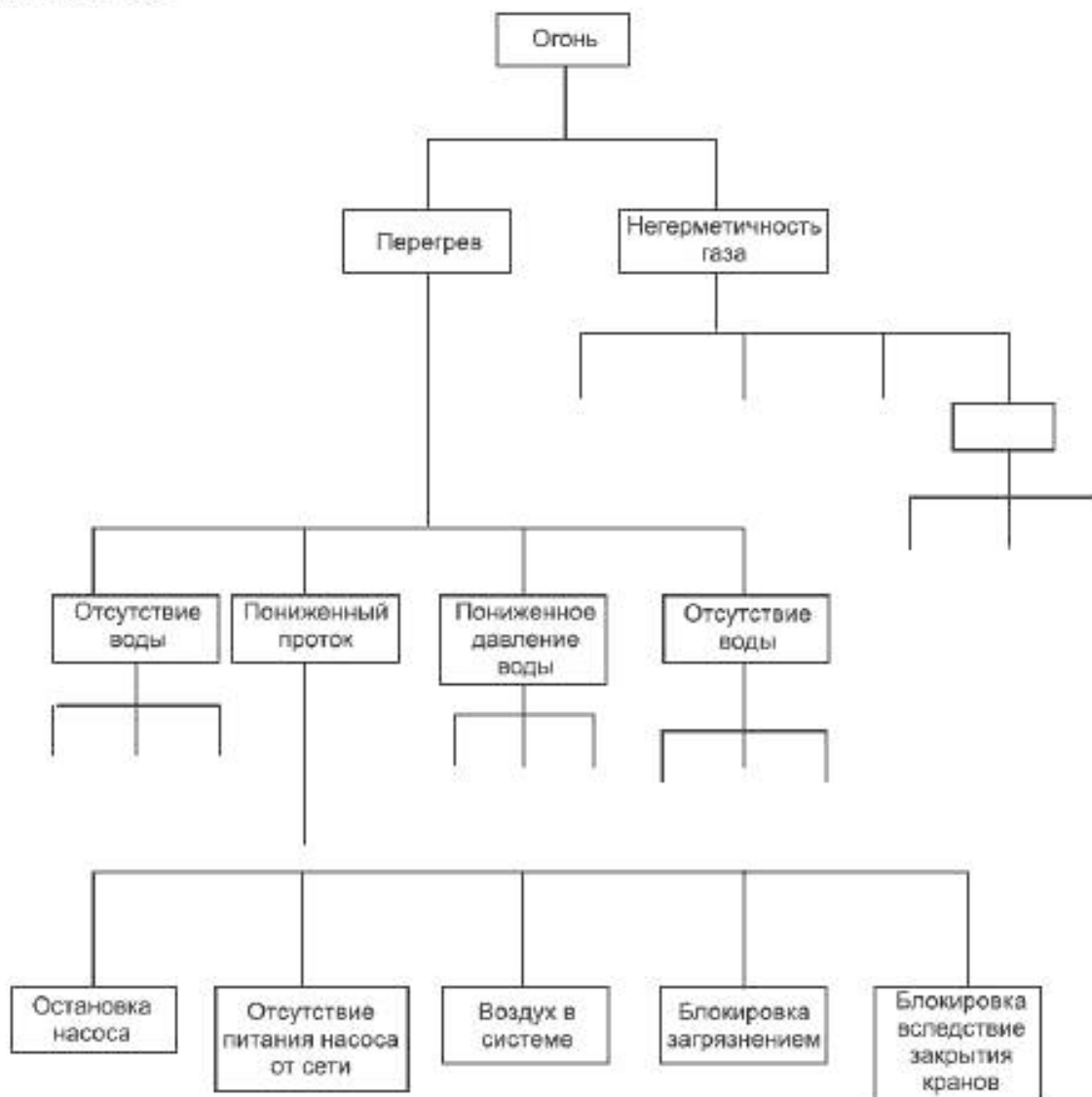
Рисунок О.1 – Схема анализа ошибок
