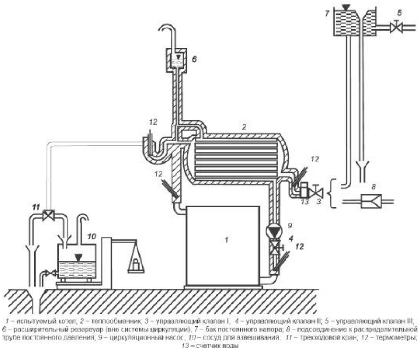
Рисунок 2 — Испытательный стенд с теплообменником
