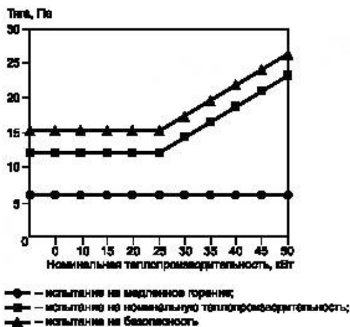
Рисунок 1 — Значения тяги в дымоходе
