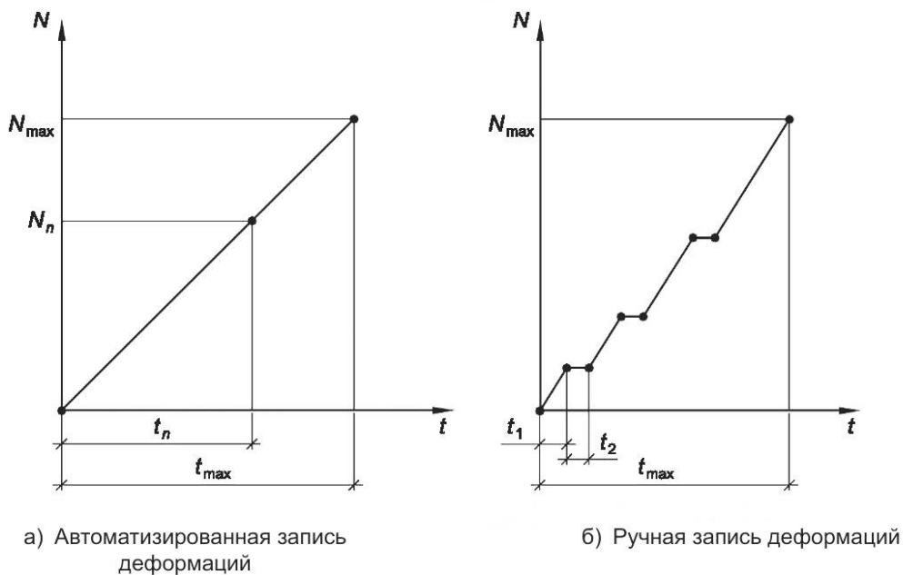
Рисунок Б.1 — Диаграмма приложения на образец непрерывно возрастающей нагрузки
