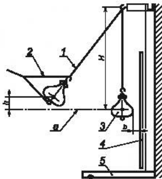
1 — стальной трос диаметром 2,5—4 мм; 2 — уздечка для подъема мешка; 3 — кожаный мешок (мягкое тело); 4 — испытуемый образец; 5 — опора; H — высота подвеса; h — высота падения мешка; a — центральная ось испытуемого образца; b — расстояние между образцом и мешком, висющим в свободном состоянии
